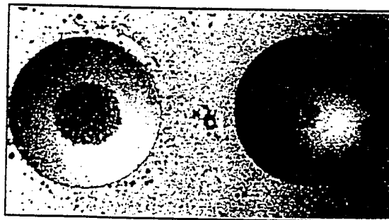
1 min. UV, 24 hr. growth
