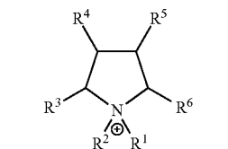
PYRROLIDIUM
