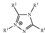
1,2,4-TRIAZOLIUM
