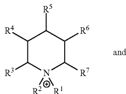
PIPERIDIUM
