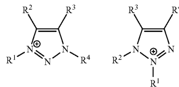
1,2,3-TRIAZOLIUM
