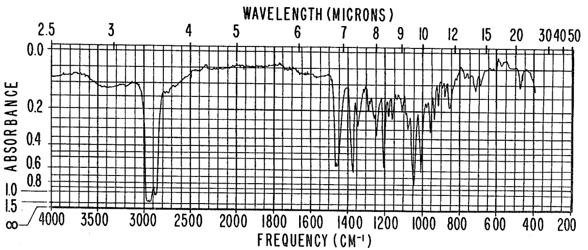
IR SPECTRUM FOR EXAMPLE X.
