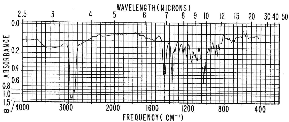
IR SPECTRUM FOR EXAMPLE VII (B).
