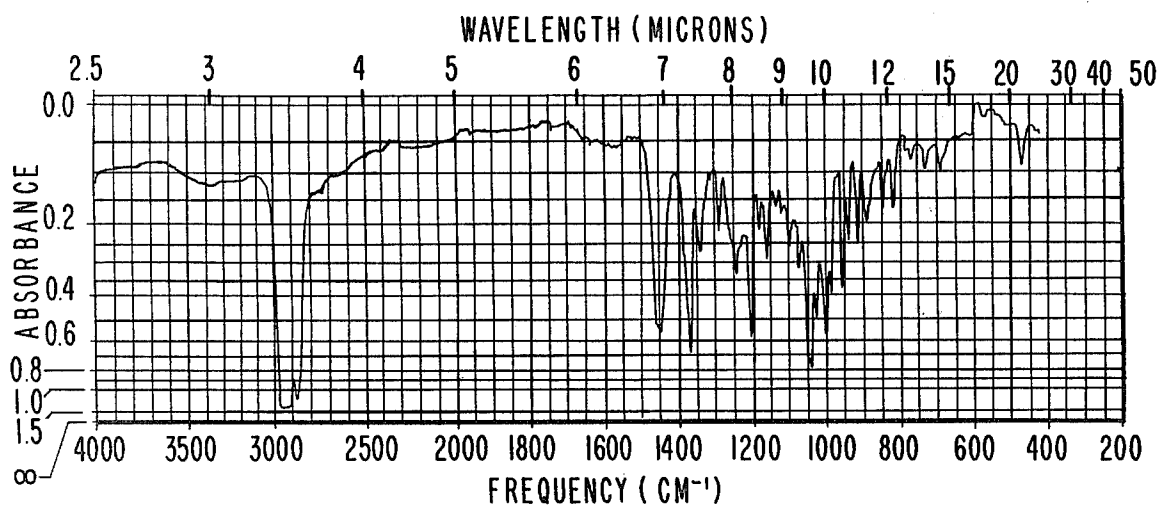
IR SPECTRUM FOR EXAMPLE IX.
