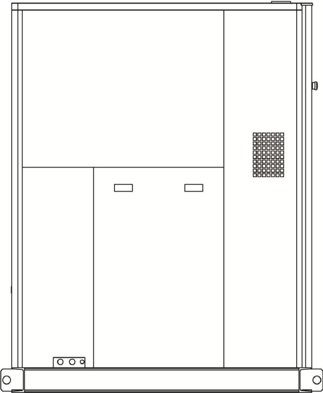
【左側視圖】
