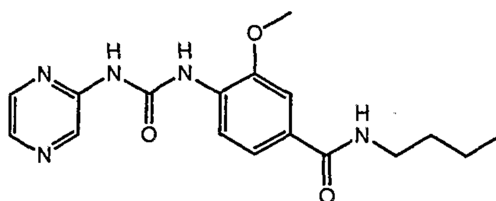
N-Butyl-3-methoxy-4-(3-pyrazin-2-yl-ureido)-benzamide
