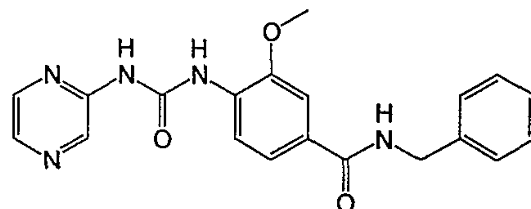
N-Benzyl-3-methoxy-4-(3-pyrazin-2-yl-ureido)-benzamide
