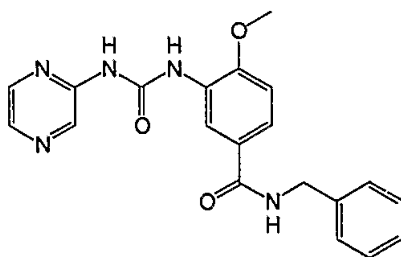
N-Benzyl-4-methoxy-3-(3-pyrazin-2-yl-ureido)-benzamide
