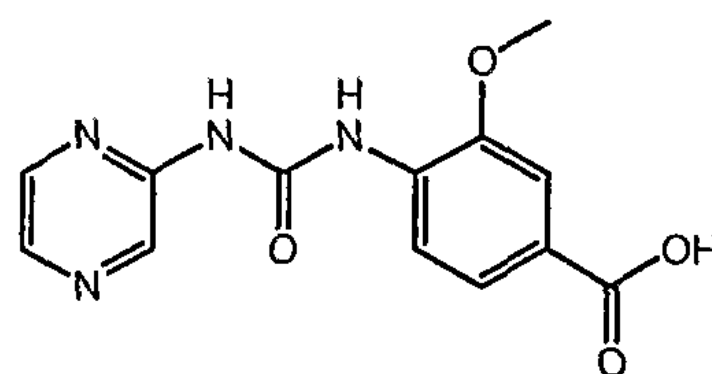
3-Methoxy-4-(3-pyrazin-2-yl-ureido)-benzoic acid
