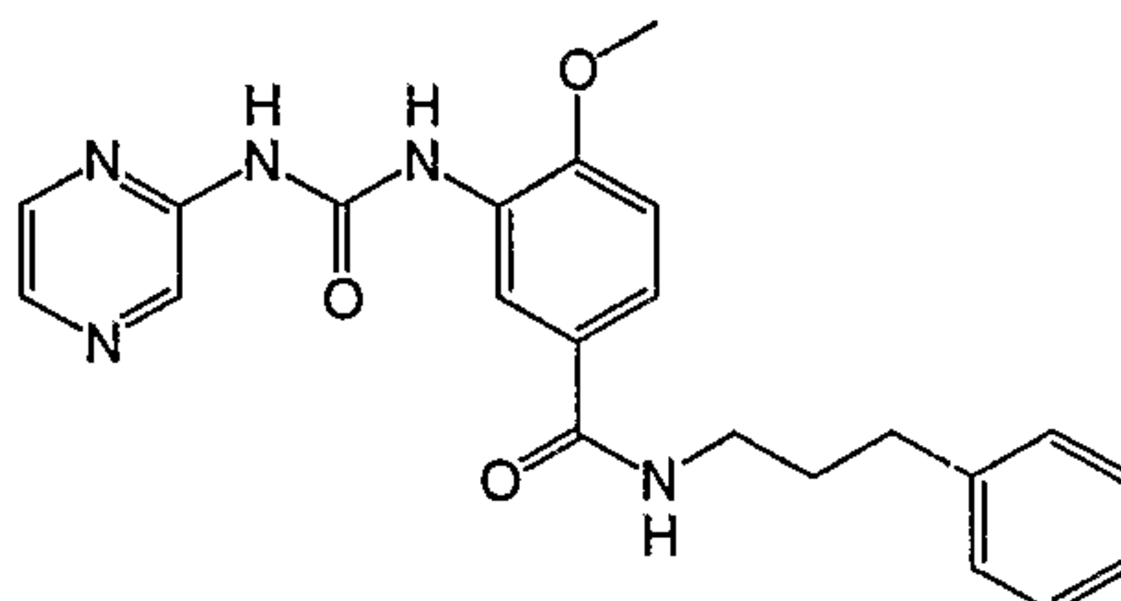
4-Methoxy-N-(3-phenyl-propyl)-3-(3-pyrazin-2-yl-ureido)-benzamide
