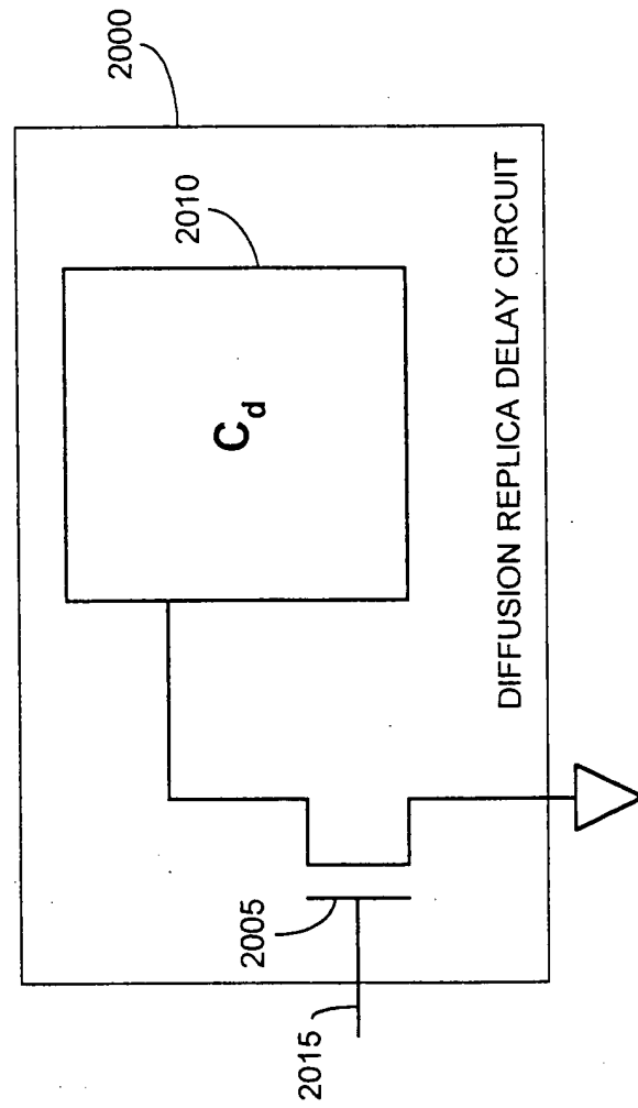
FIG. 20
