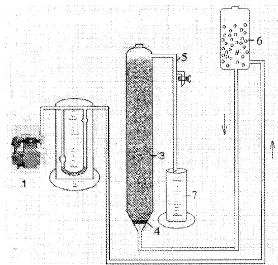
Fig. 1. Shema instalației pentru oxidarea nitriților în condiții dinamice 1 – pompă de aer, 2 – contor de aer, 3 – coloană cu cărbune activ, 4 – filtru de sticlă, 5 – ieșire pentru colectarea probelor, 6 – rezervor pentru apa ce conține ioni de nitriți, 7 – rezervor pentru apa purificată.
