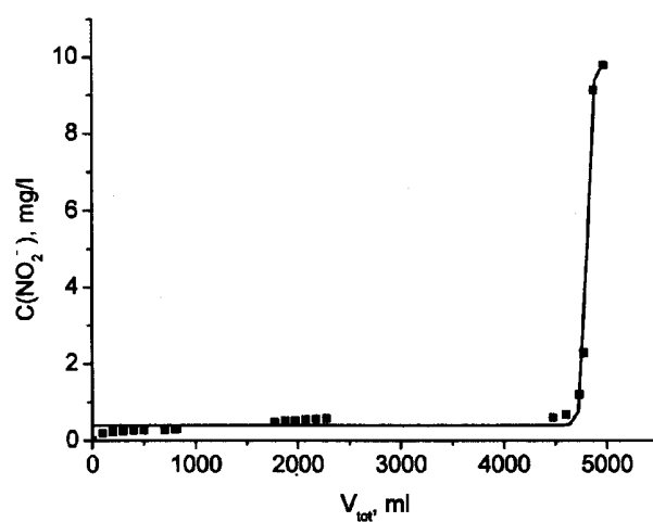
Fig. 2. Curba dinamică de oxidare a nitriților prin aerare.
