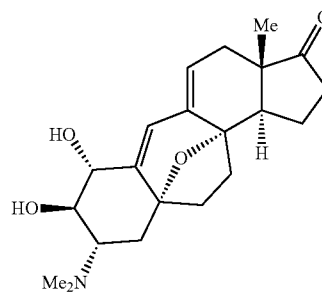
Cortistatinone 8
