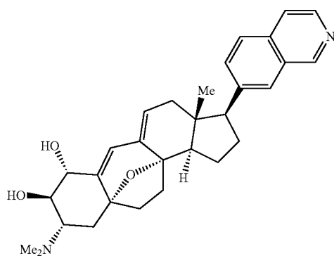
Cortistatin A (1)
