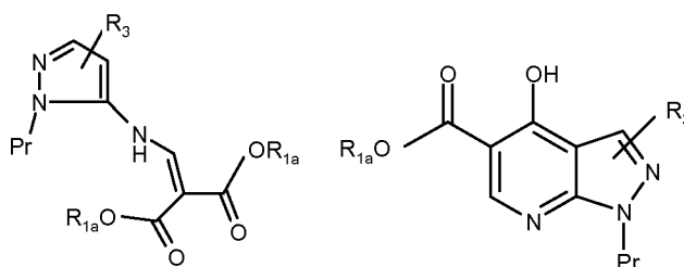
Formula LI
