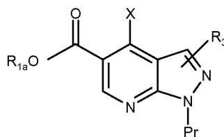
Formula LIII
