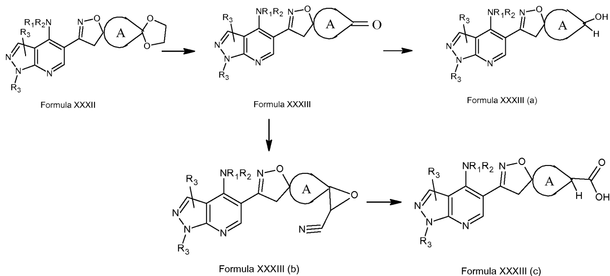
Scheme VI
