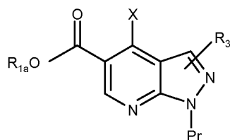
Formula LIII
