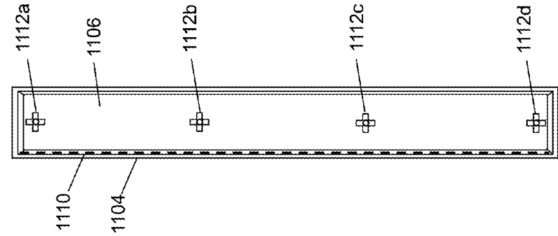
FIG. 11E (End View)
