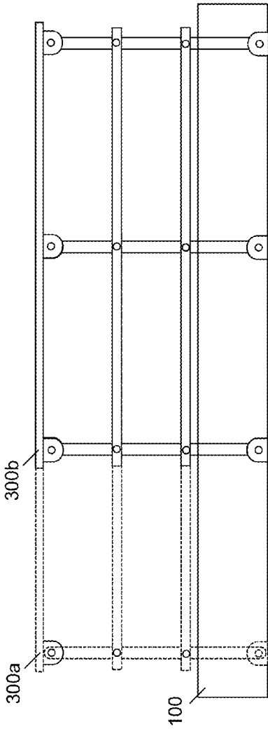
FIG. 10E (Side View)
