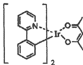
Ir(ppy) 2 (acac)
