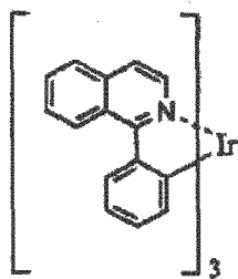
Ir(piq) 3
