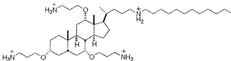
CSA-131 CLogP: 7.344
