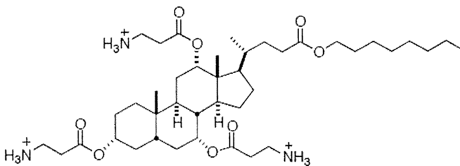
CSA-44 CLogP: 6.351
