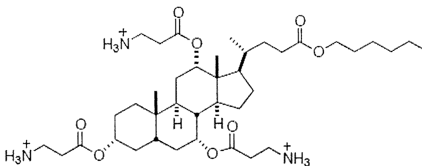
CSA-142 CLogP: 5.293
