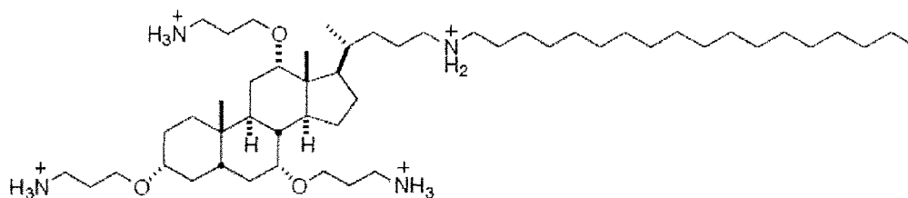
CSA-132 CLogP: 10.518
