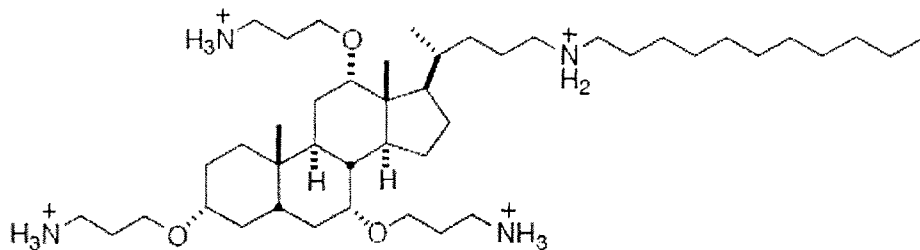
CSA-137 CLogP: 6.815
