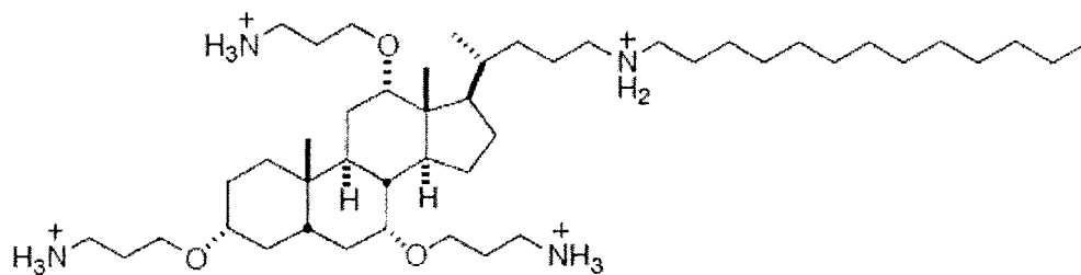
CSA-138 CLogP: 7.873
