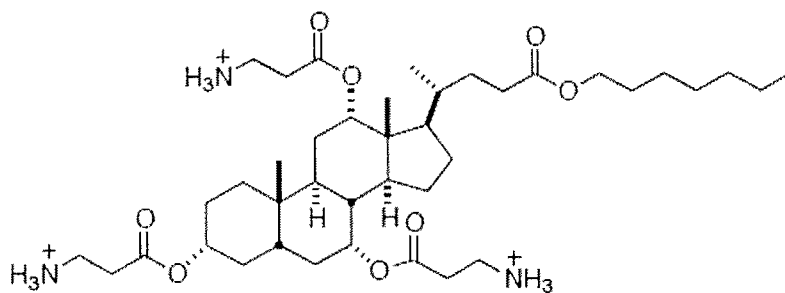
CSA-146 CLogP: 5.822
