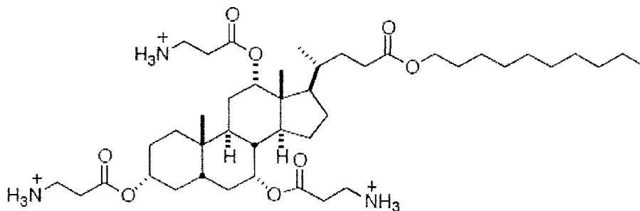
CSA-144 CLogP: 7.409
