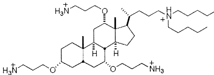
CSA-90 CLogP: 6.0858
