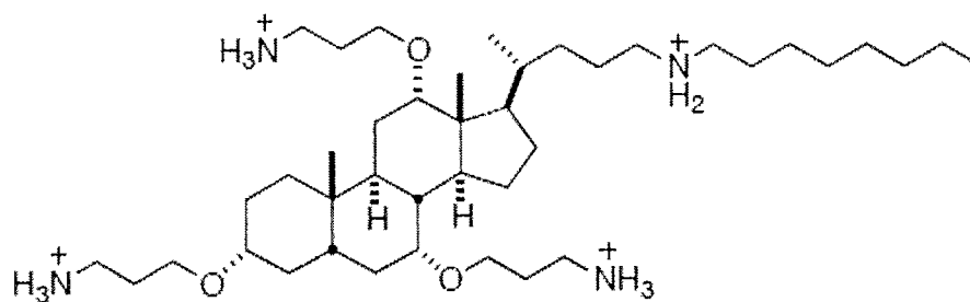
CSA-13 CLogP: 5.228
