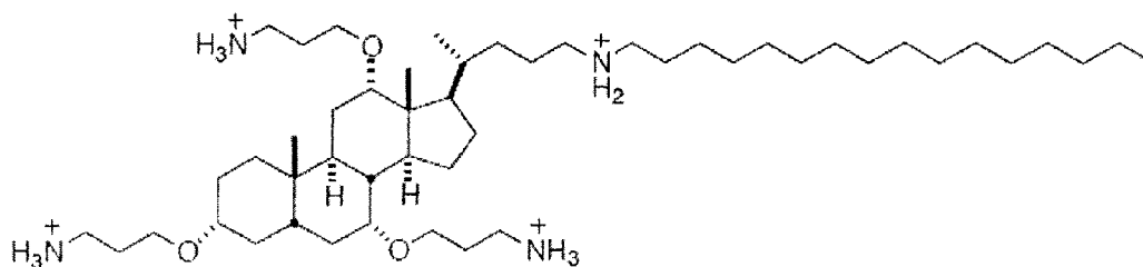
CSA-135 CLogP: 9.46
