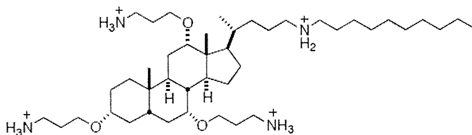
CSA-136 CLogP: 6.286
