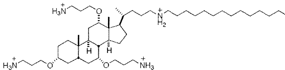
CSA-134 CLogP: 8.402
