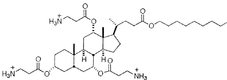
CSA-145 CLogP: 6.88
