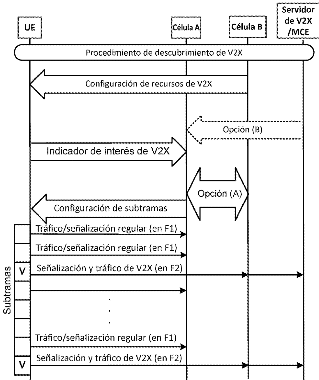
Multiplexación de tiempo/subtramas entre F1 y F2
