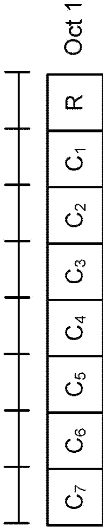
Elemento de control de MAC de activación/desactivación de ejemplo de un octeto
