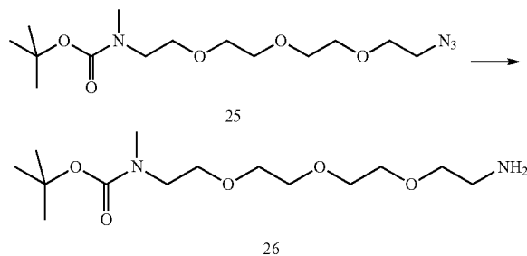
Compound 26 tert-Butyl (2-{2-[2-(2-aminoethoxy)ethoxy] ethoxy}ethyl)methylcarbamate
