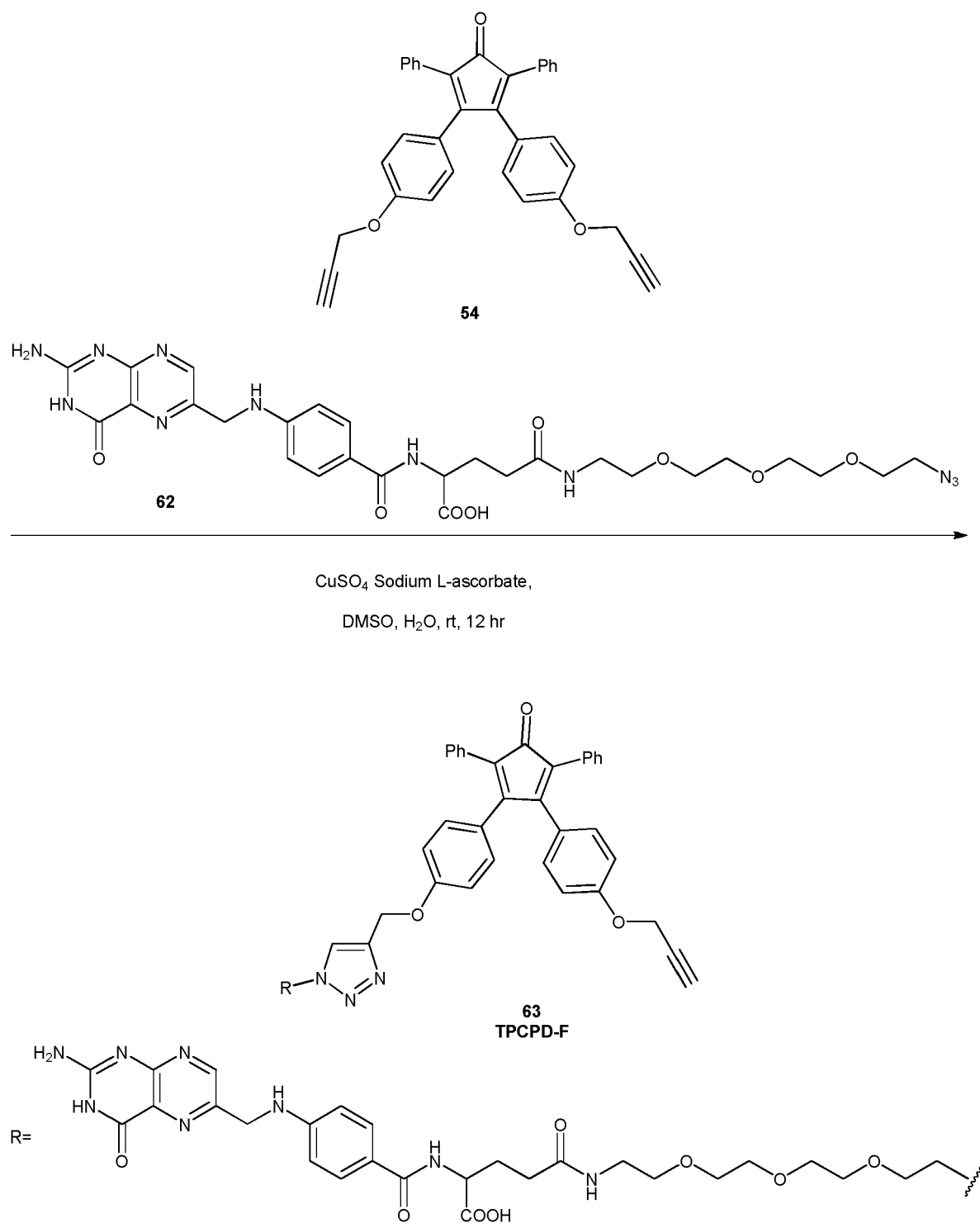
Scheme 17.
