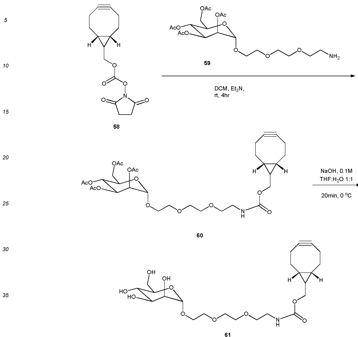
Scheme 16—cont'd.
