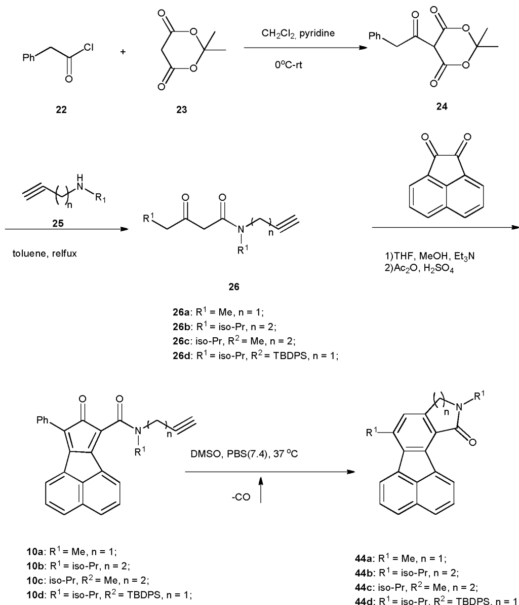
Scheme 14.
