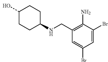
ambroxol
