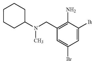
bromhexine
