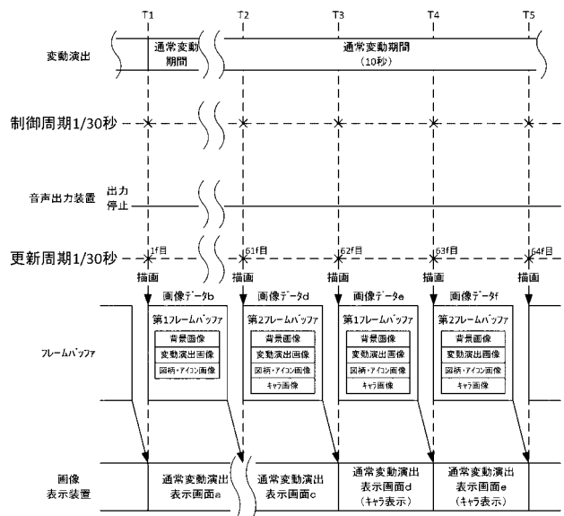
キヤ作用変化パターン01のタイミングチャート1
