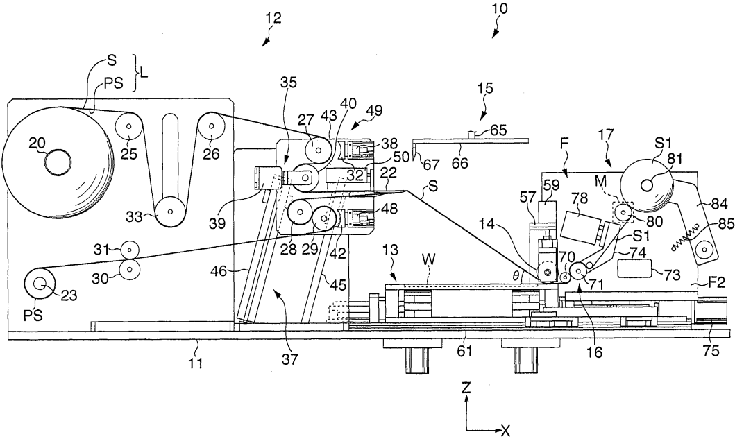
도면1
