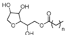
Sorbitan Ester n = 6-12
