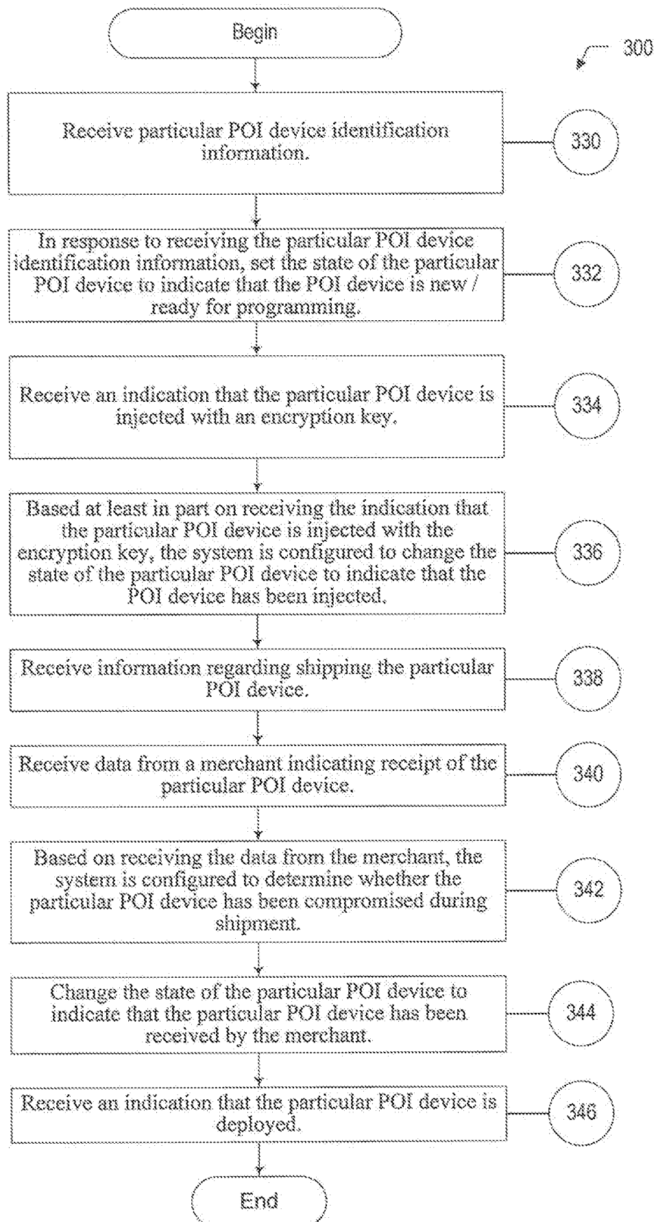
FIG. 3 EXEMPLARY POI HANDLING PROCESS
