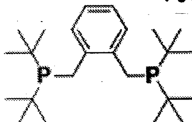
1,2-bis(di-tertbutylphosphinomethyl)benzen
