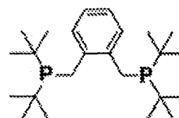
(P-P) Ligand
