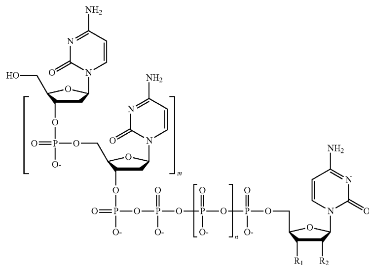
(dCp)_m-(PO_4)_n-dC
