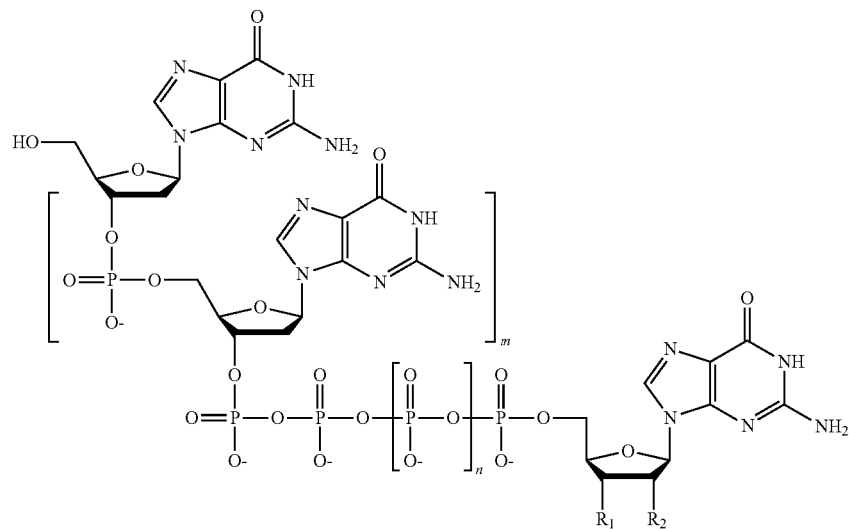
(dGp)_m-(PO_4)_n-dG
