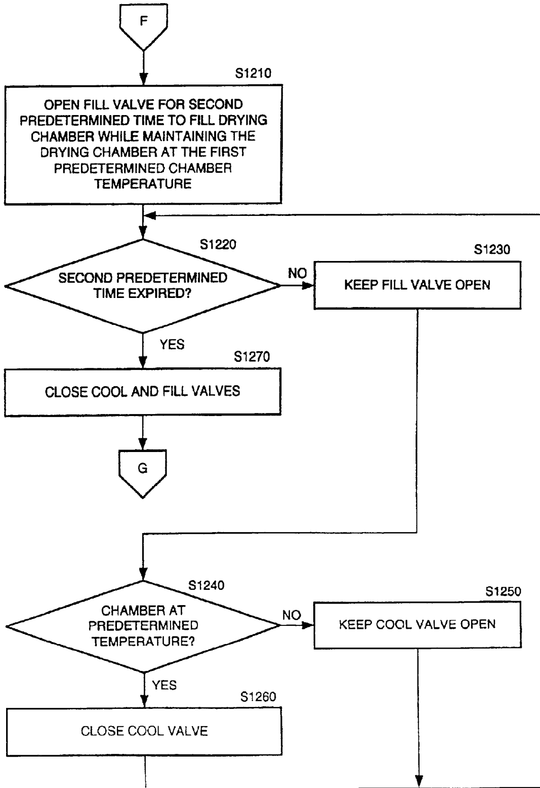
FIG. 15D
