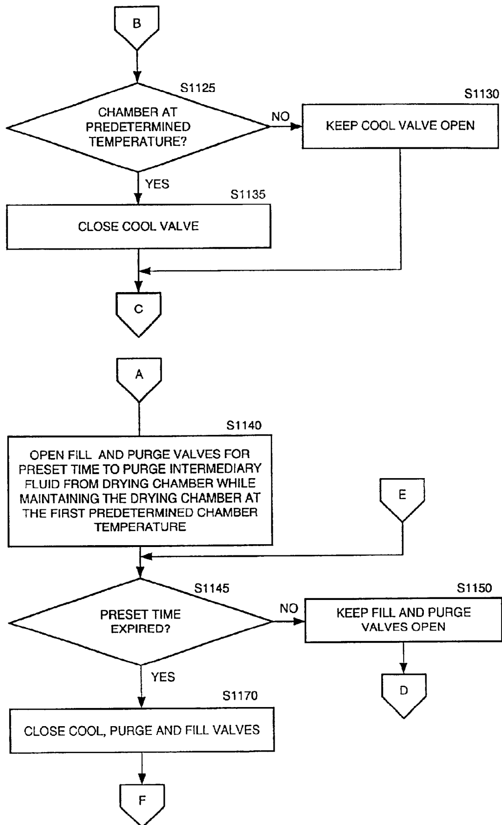
FIG. 15B
