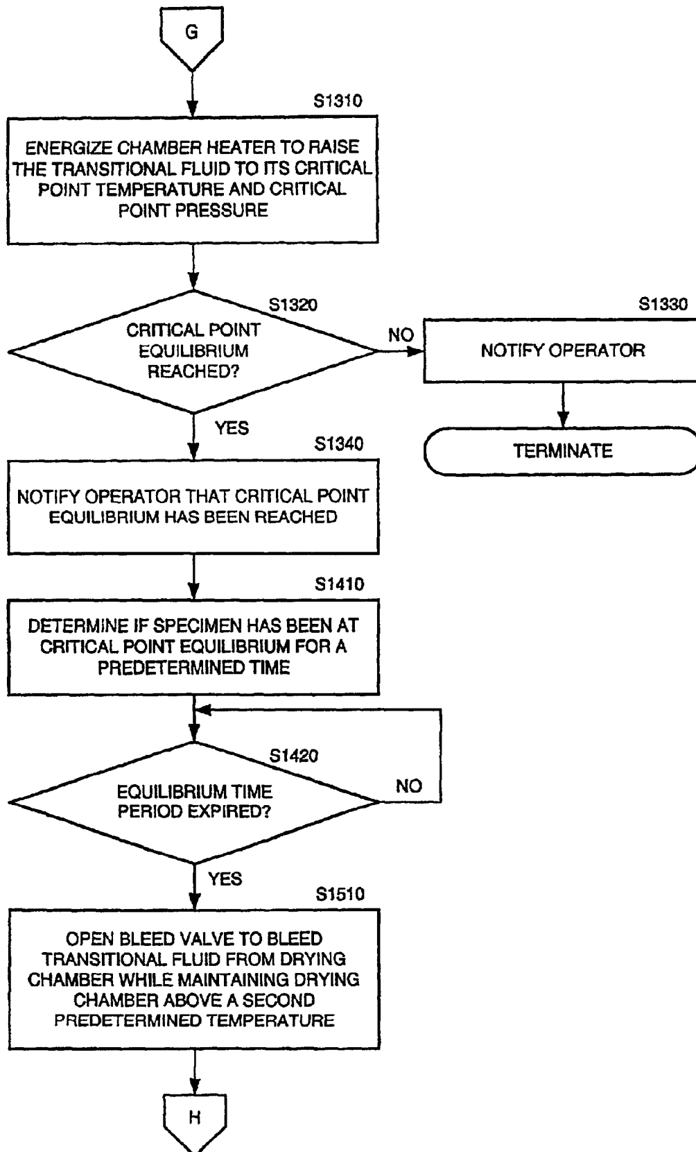
FIG. 15E
