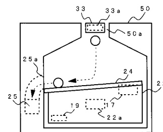
(A) 可変入球装置閉鎖中
