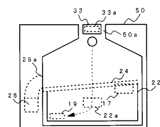
(B) 可変入球装置開放中
