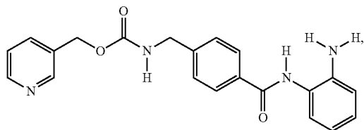
MS-275
