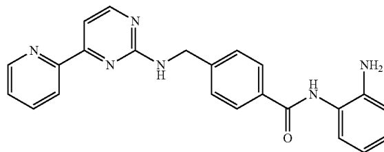
N-(2-Aminophenyl)-4-[[[4-pyridin-3-ylpyrimidin-2-yl]amino]methyl]benzamide
