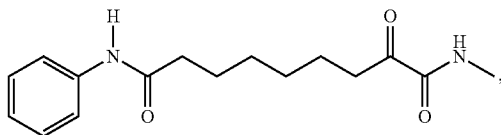
alpha-cétoamide
