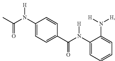
Cl-994
