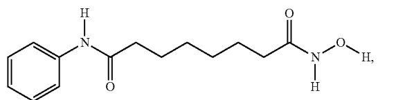
SAHA
