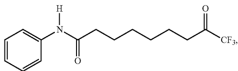
Trifluorométhyl cétone
