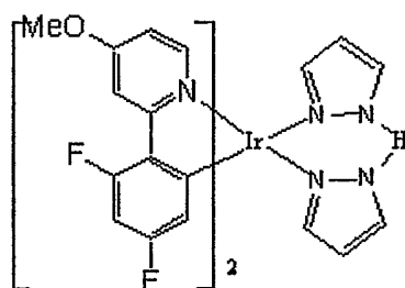
( MeOfppy ) 2 Ir(pz 2 H)
