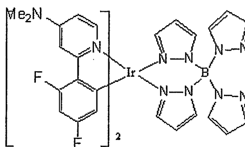
( dmaffppy ) 2 Ir(pz 2 Bpz 2 )
