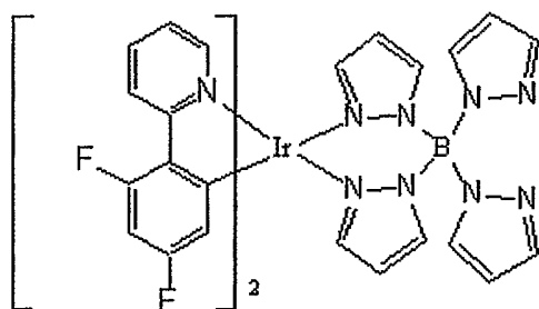
( fppy ) 2 Ir(pz 2 Bpz 2 )
