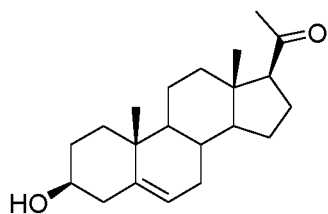
Pregnenolone
