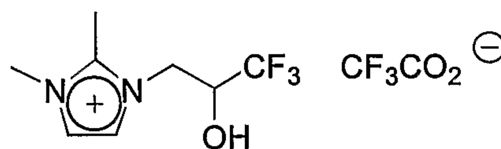
Fluoro alcohol IL 1
