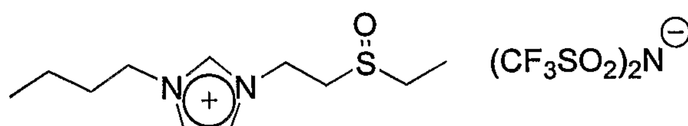
Sulfoxide IL 2
