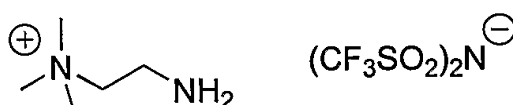
Amine IL 7
