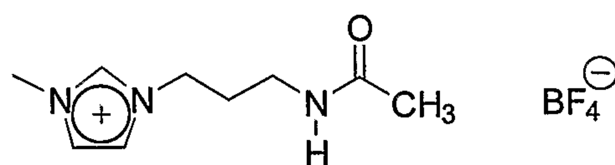
Acyclic amide IL 1
