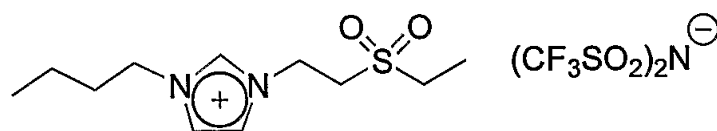
Sulfone IL 2
