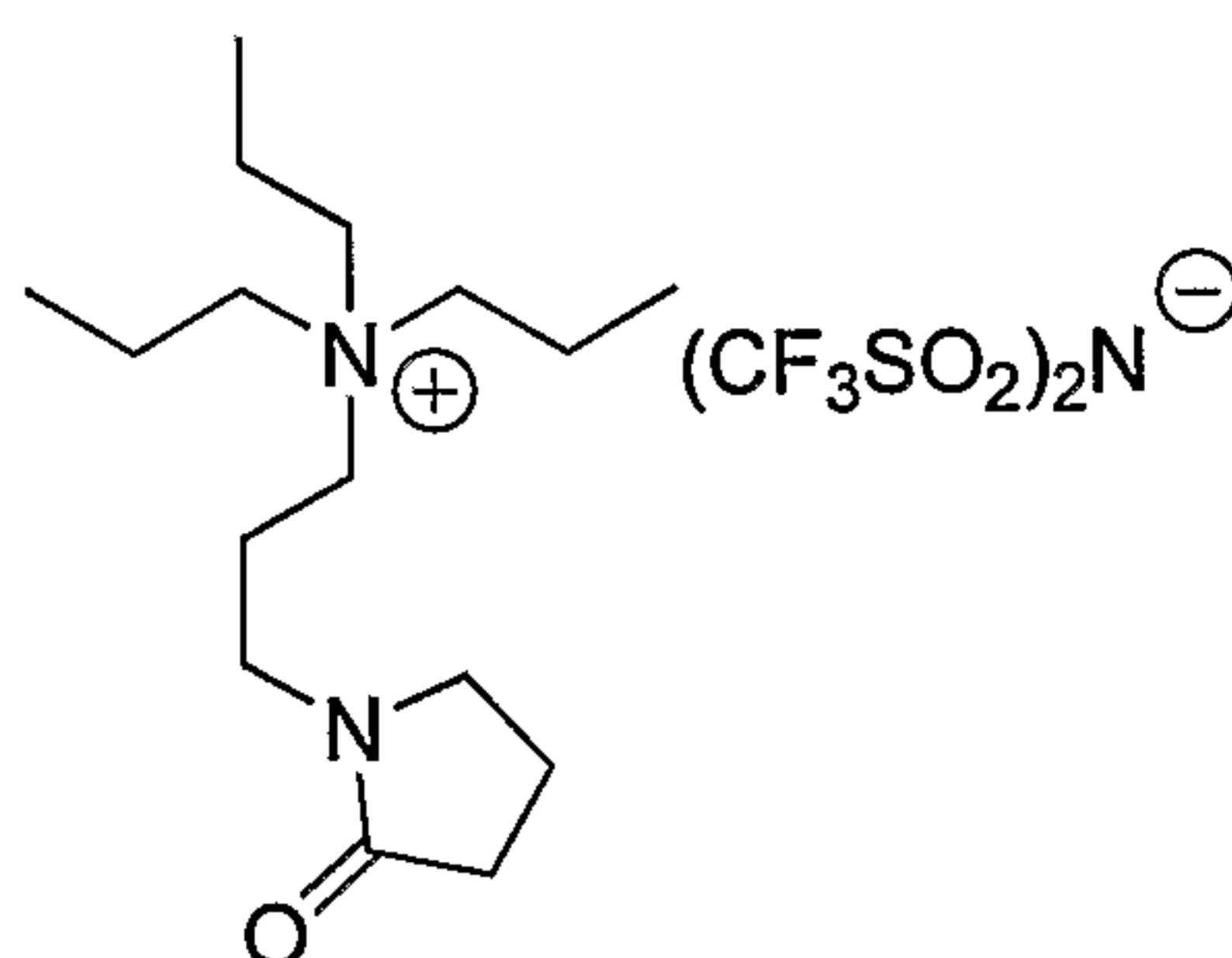
Cyclic amide IL 2
