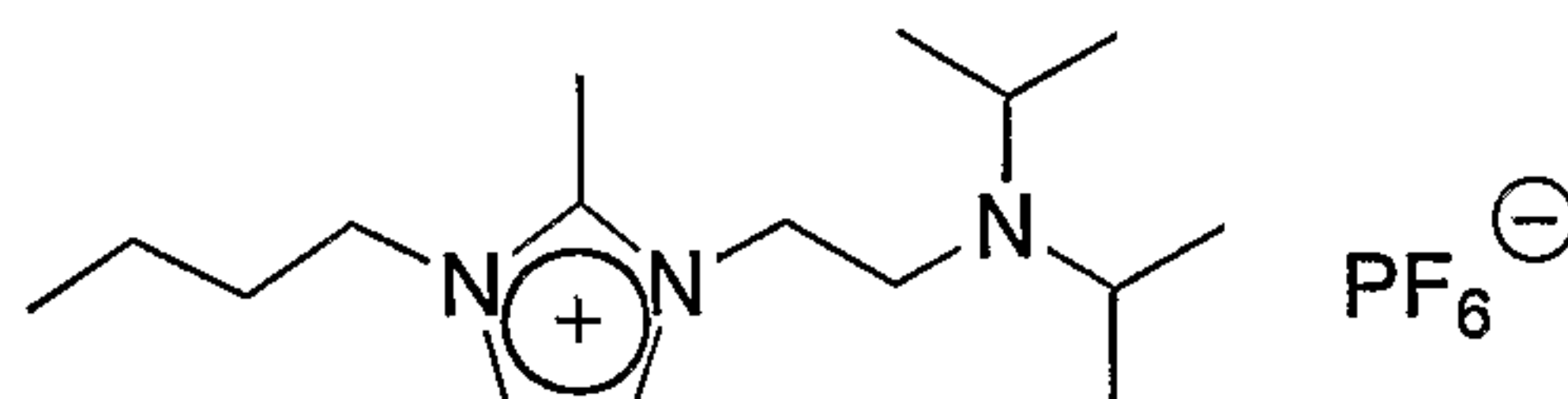
Amine IL 2
