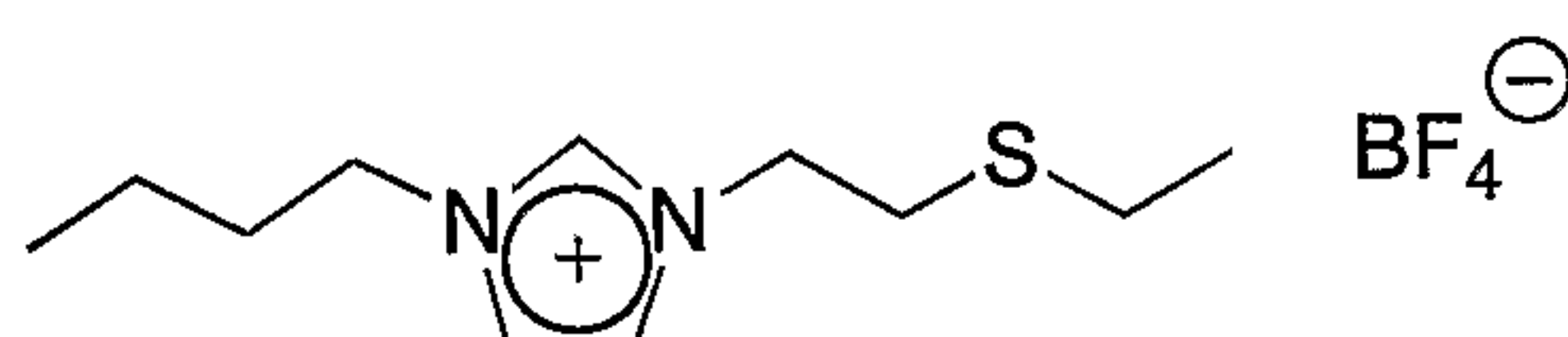
Thioether IL 1
