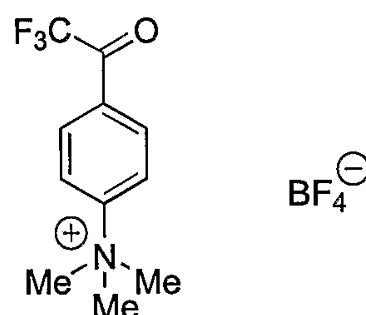
Fluoro ketone IL 1
