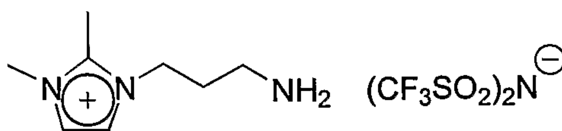
Amine IL 1
