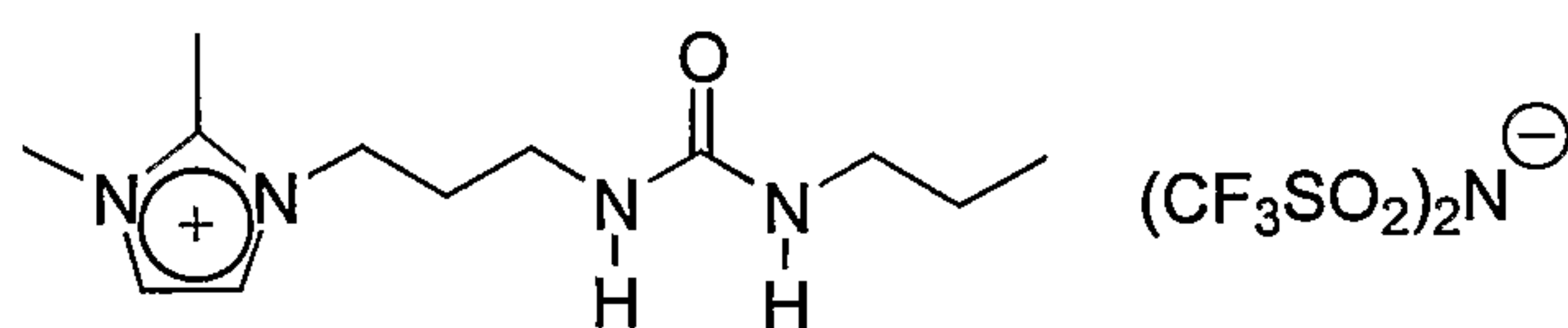
Acyclic amide IL 3
