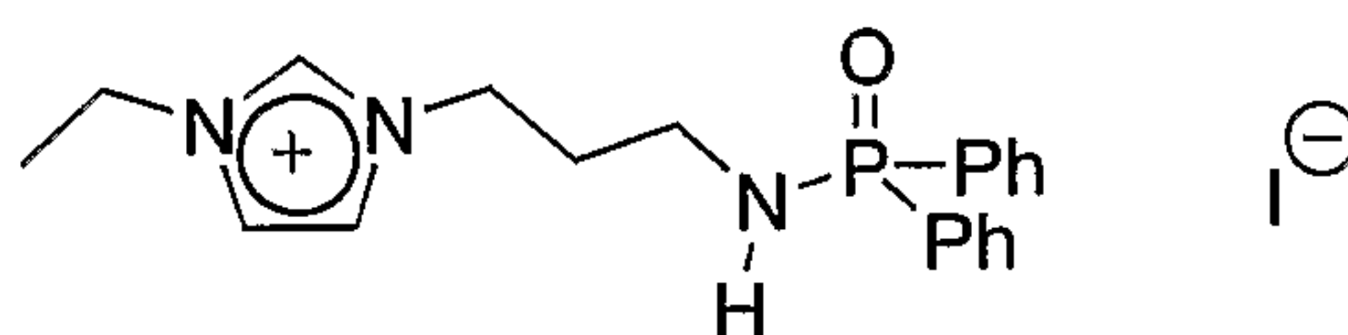
Phosphoramidate appended IL 1
