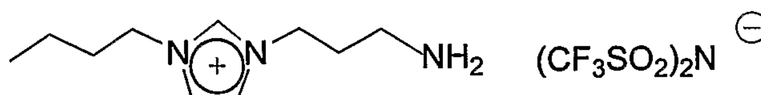
Amine IL 3
