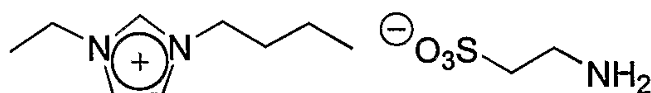
Amine IL 5
