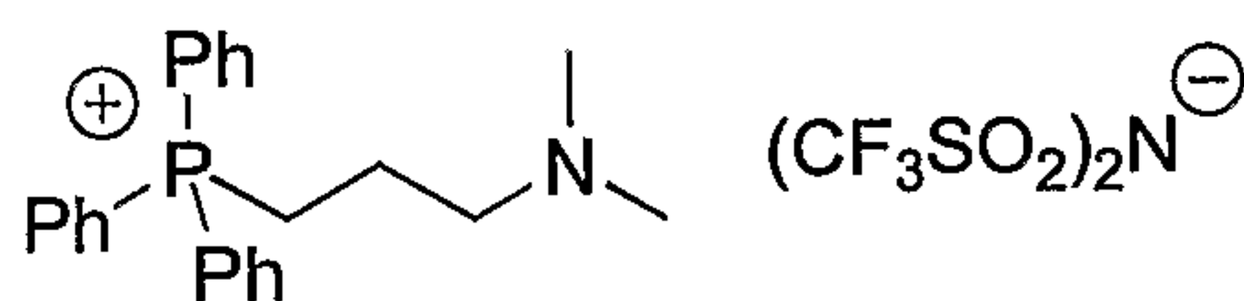
Amine IL 4
