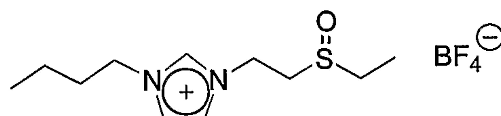
Sulfoxide IL 1
