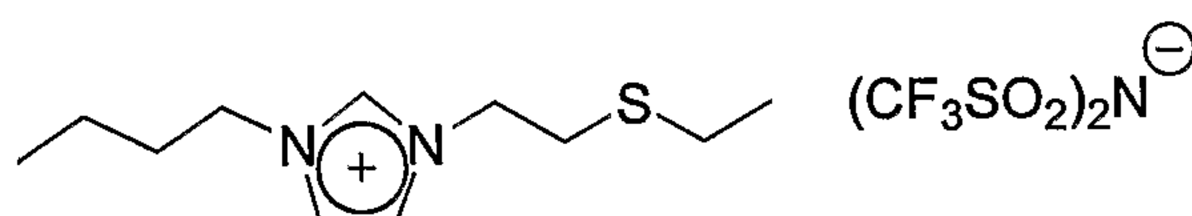
Thioether IL 2
