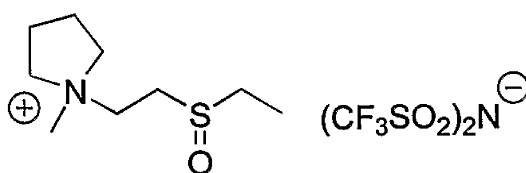
Sulfoxide IL 5
