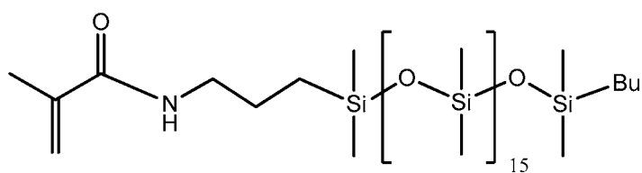
Ma1D15
