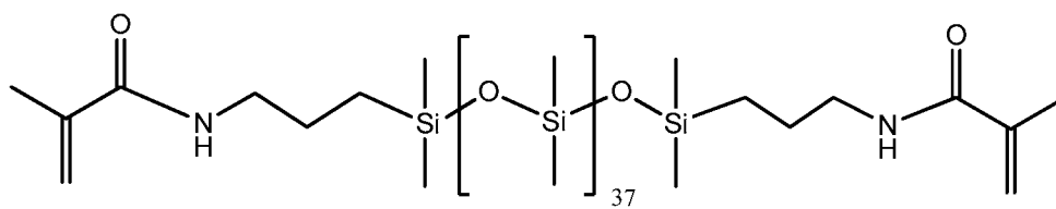
Ma2D37
