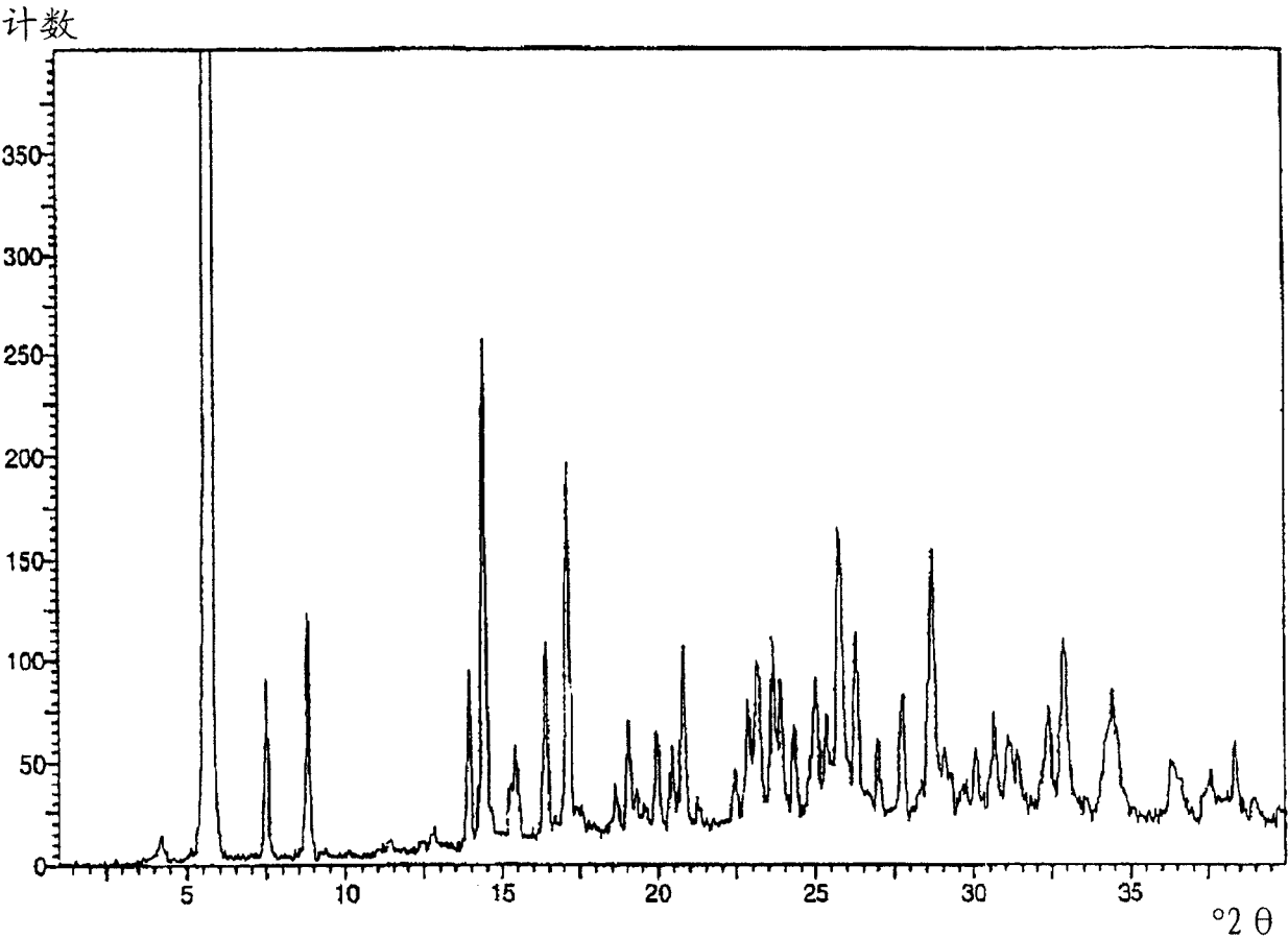
图4 用可调节的狭缝测量的依美拉唑钠盐修饰物C的 X线粉末衍射图, 图3的放大版
