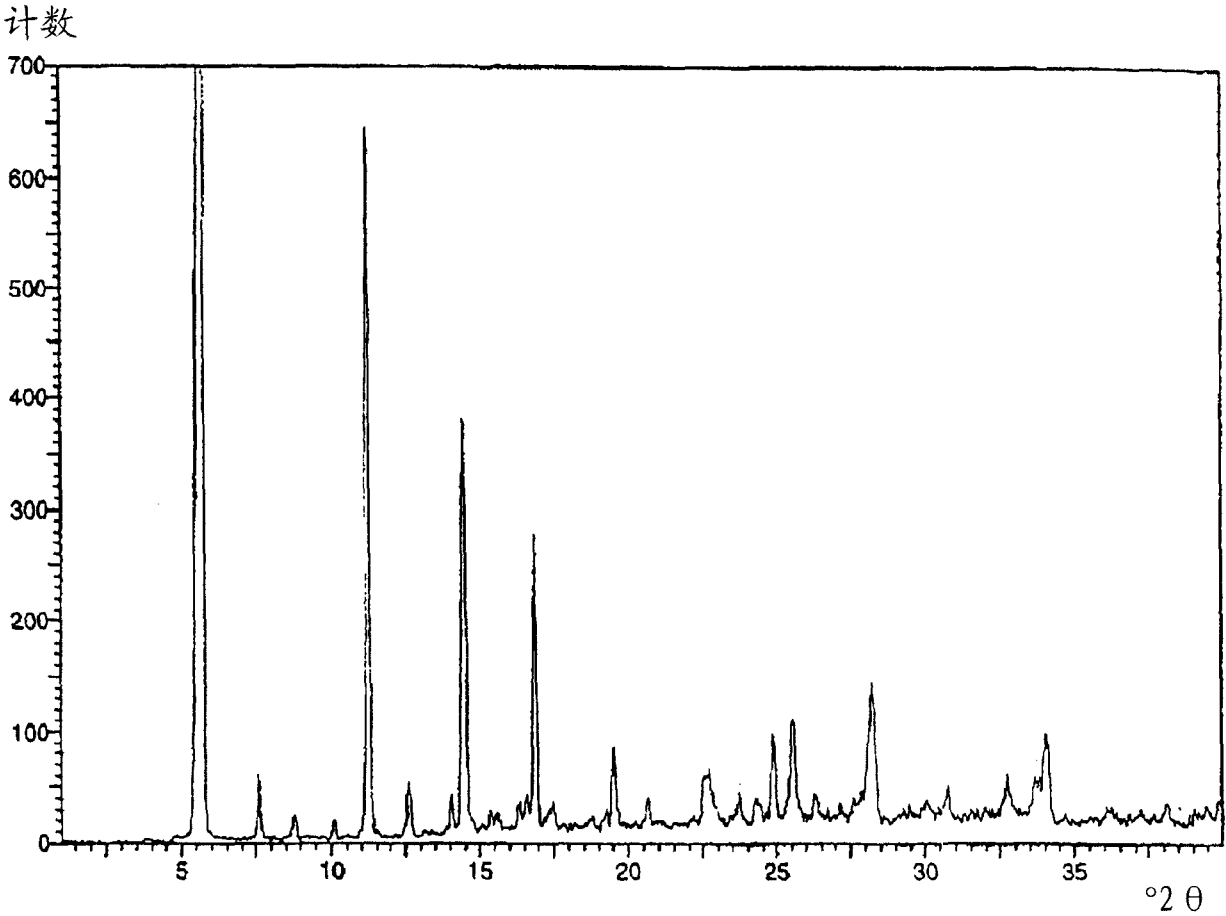
图2 用可调节的狭缝测量的依美拉唑钠盐修饰物C的X线粉末衍射图, 图1的放大版
