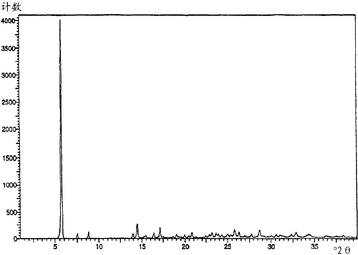
图3 用可调节的狭缝测量的依美拉唑钠盐修饰物E的X线粉末衍射图
