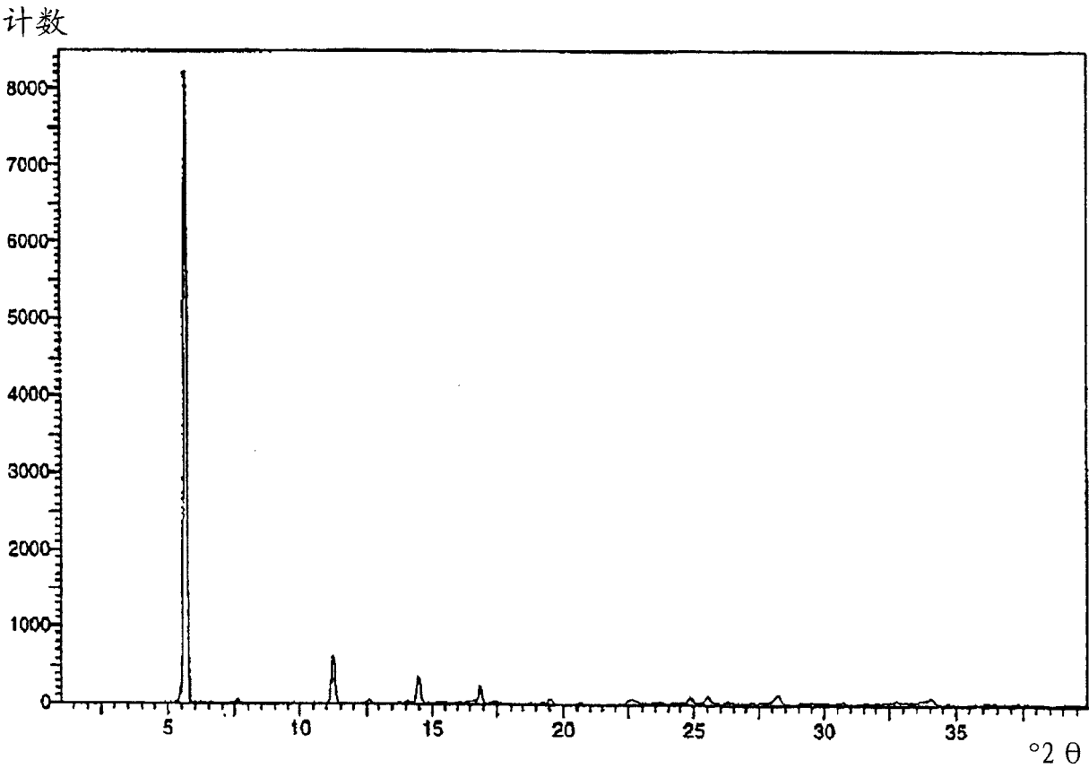
图1 用可调节的狭缝测量的依美拉唑钠盐修饰物C的X线粉末衍射图
