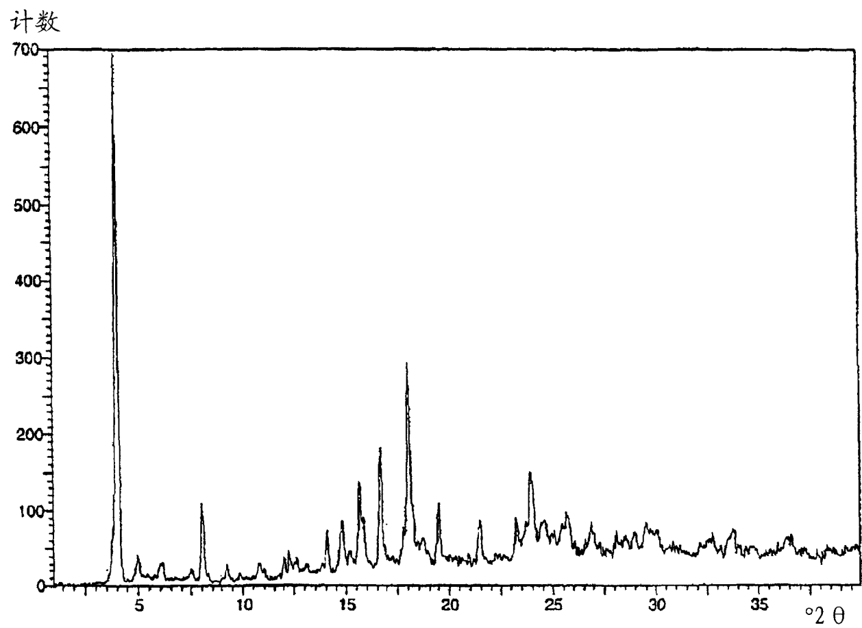
图5 用可调节的狭缝测量的依美拉唑钠盐修饰物H的X线粉末衍射图
