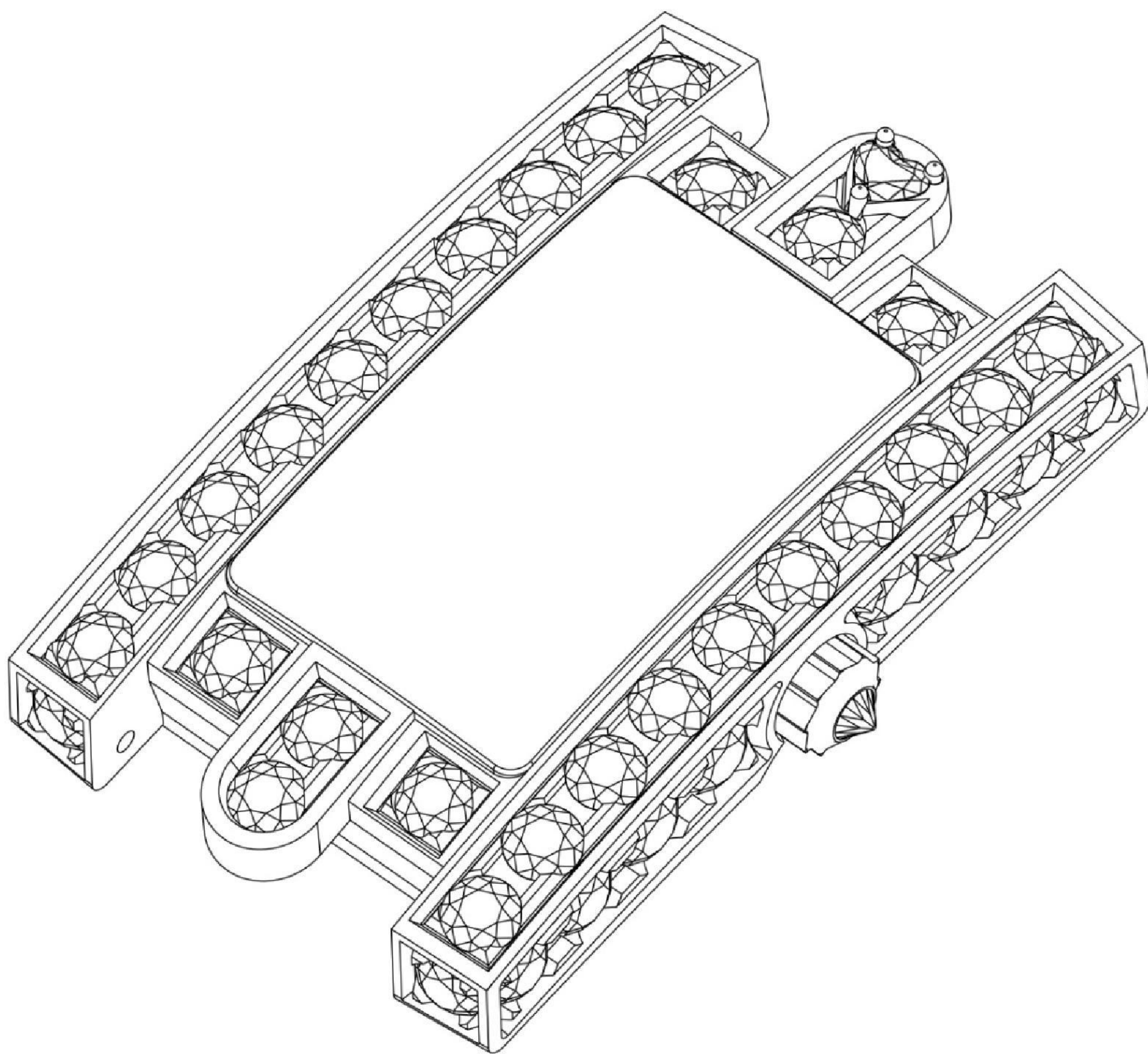
【立體圖1】
