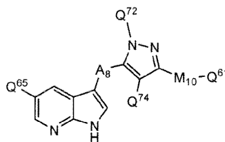
Formula IIg.
