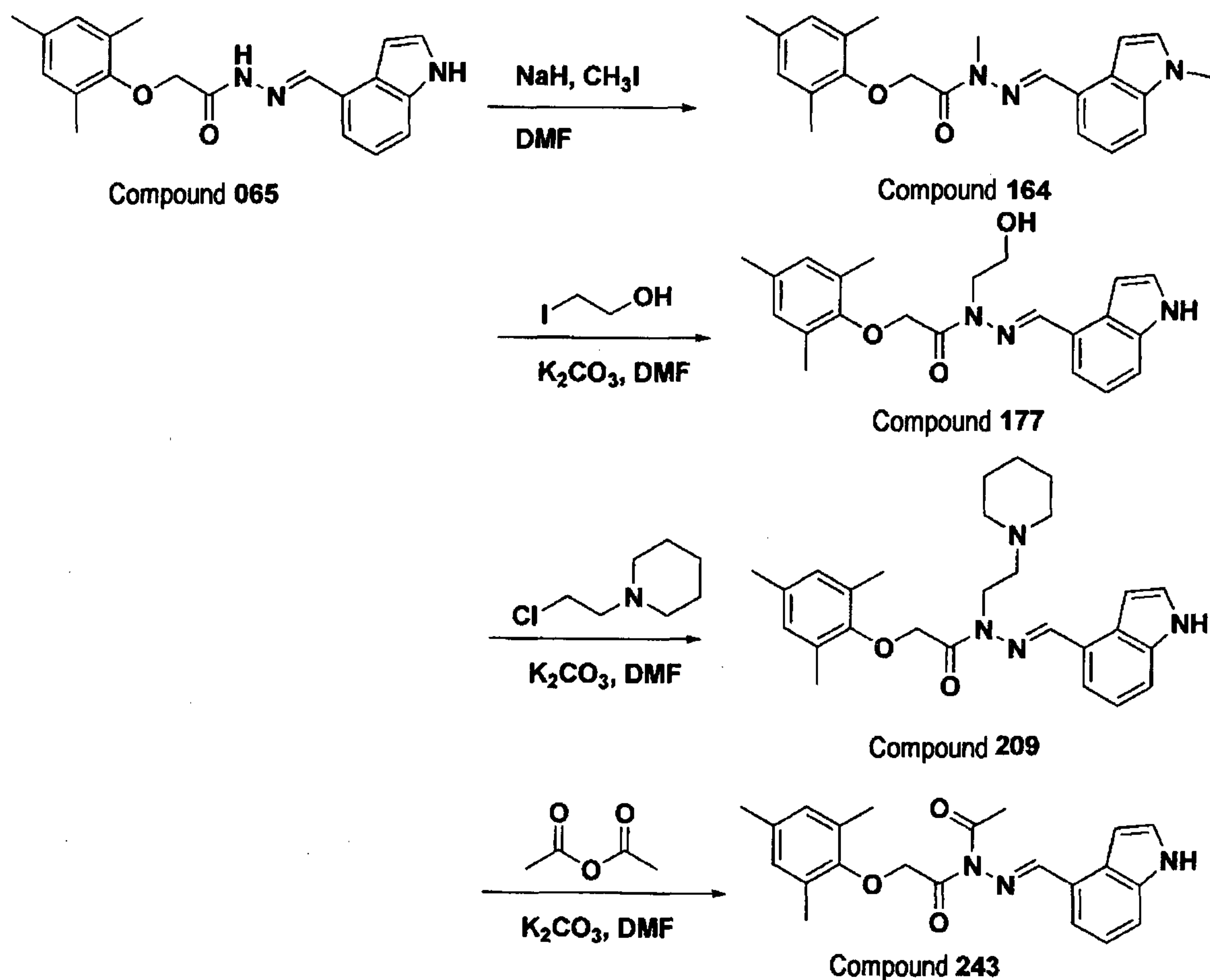
[Scheme 3]
