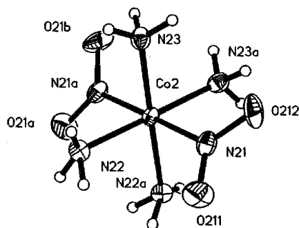
Fig. 1. Structura cationului complex al compusului I
