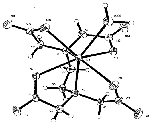
Fig. 2. Structura anionului complex al compusului I
