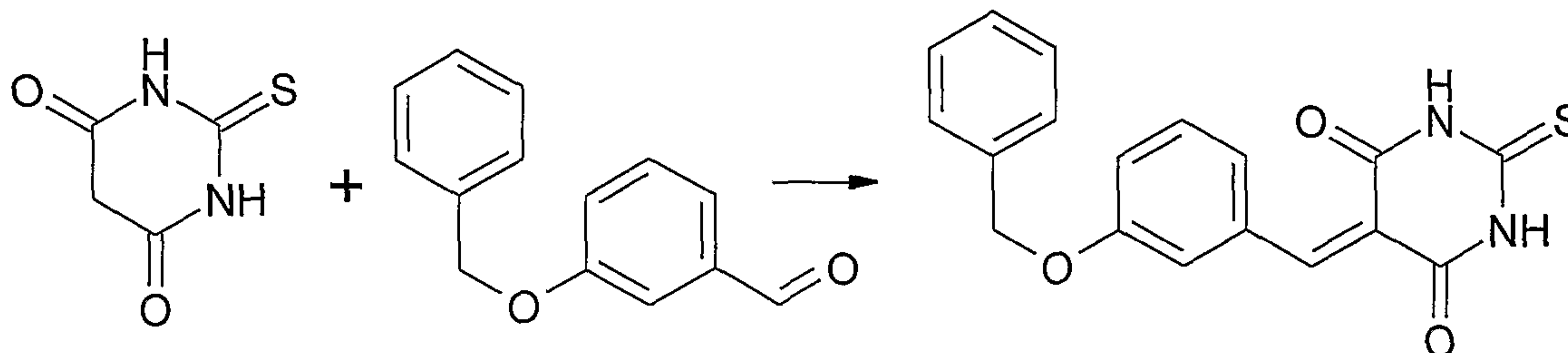
Scheme 13 - Ismail et al., 1997
