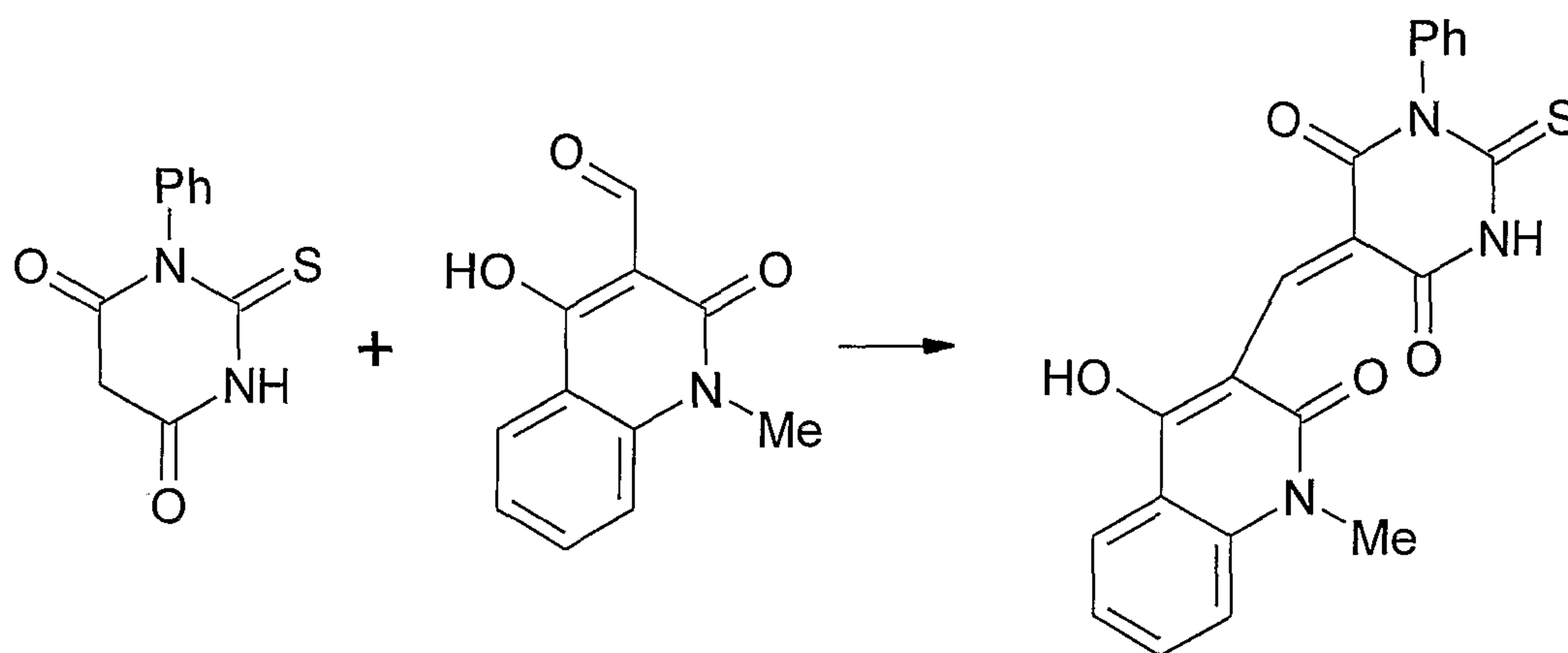
Scheme 13 - Ismail et al., 1997
