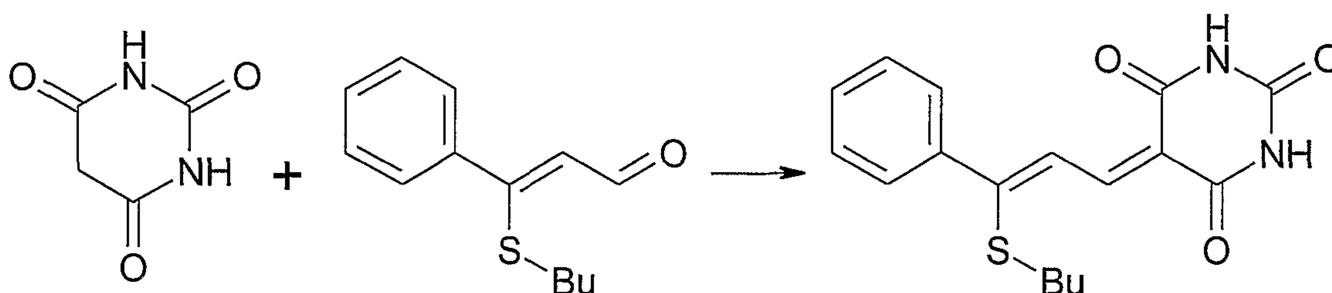
Scheme 2 - Andreani et al., 1996
