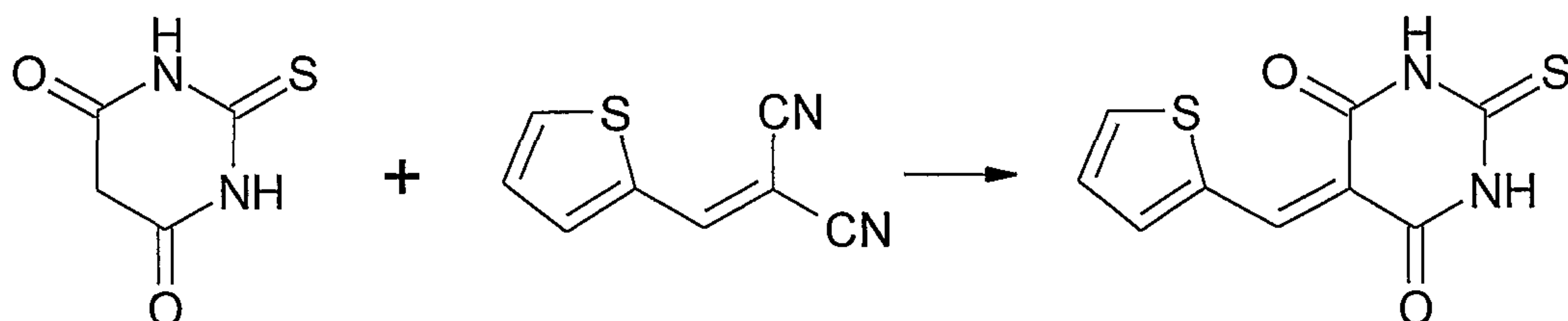
Scheme 15 - Abdel-Latif, 1991
