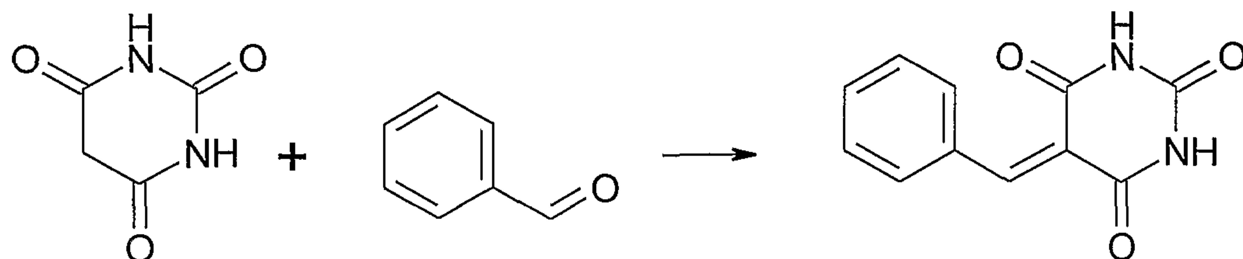
Scheme 5 - Rao et al., 1993
