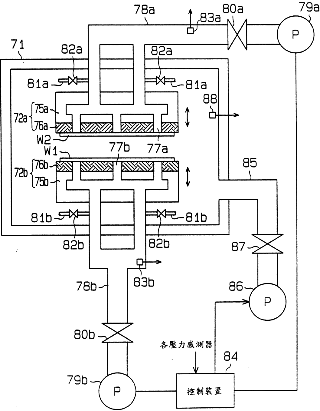
說明真空環境中的基板吸著的概略圖
