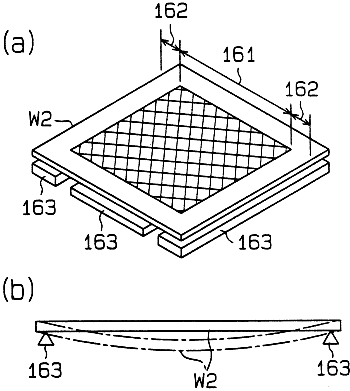
基板搬送及基板發生翹曲的說明圖
