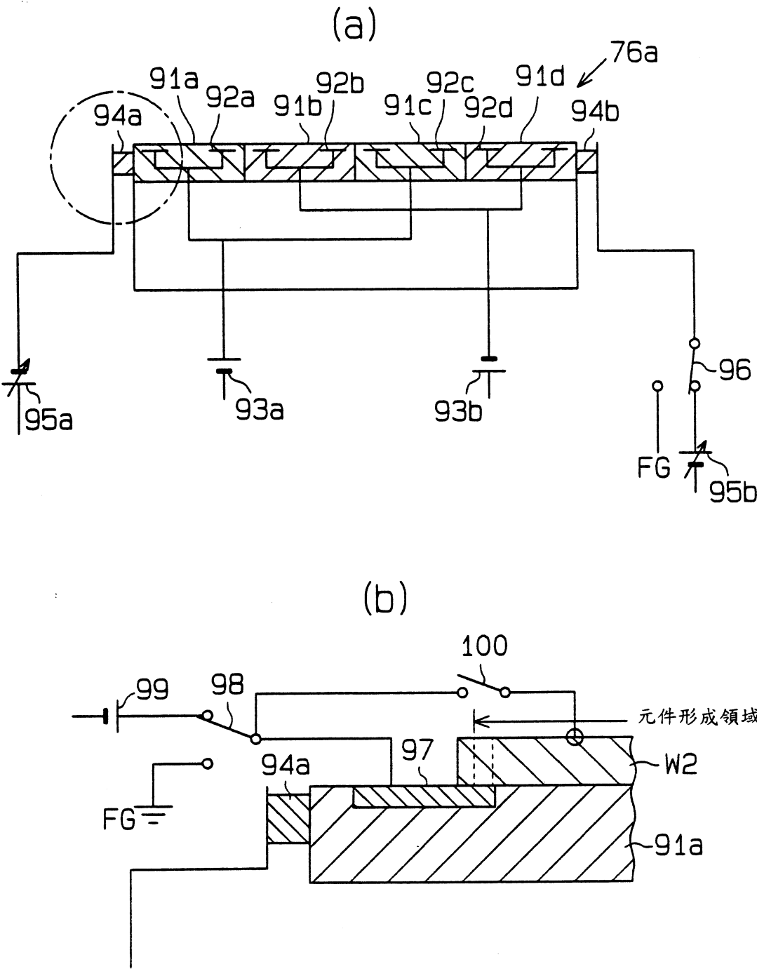
靜電夾箱器之說明圖
