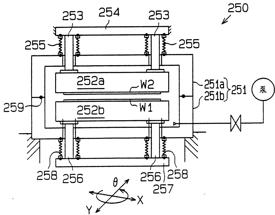
對於第31圖之習知例的概略構成圖
