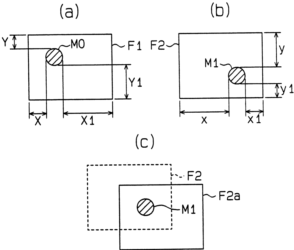
合對位置標記之說明圖
