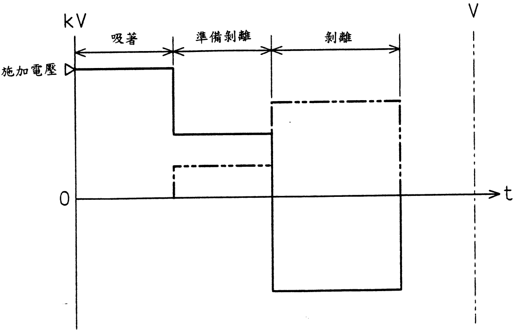
施加於靜電夾箱器之電壓的波形圖
