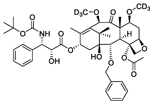
cabazitaxel-7,10-d6
