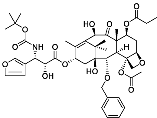
Milataxel
