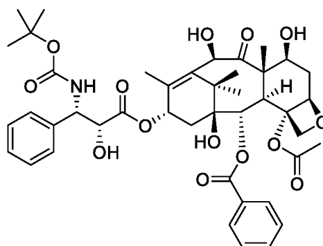
Docetaxel (Taxotere)
