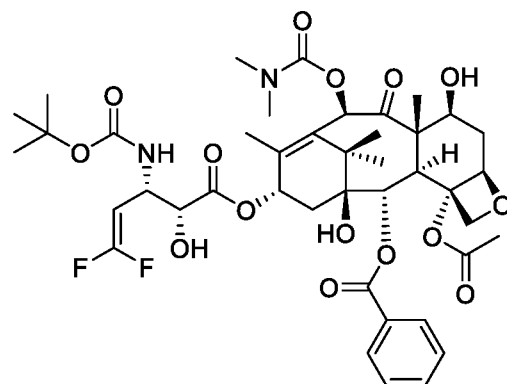
SB-T-12854
