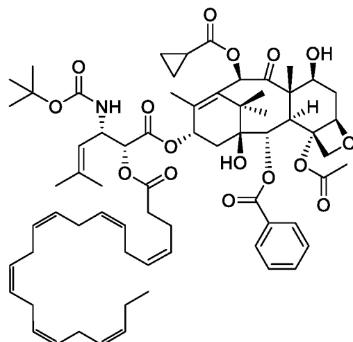
DHA-SB-T-1214
