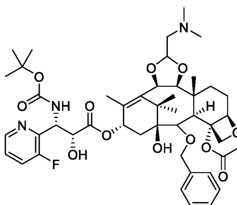
Tesetaxel
