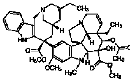
Vinorelbine
