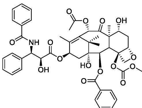
BMS-188797
