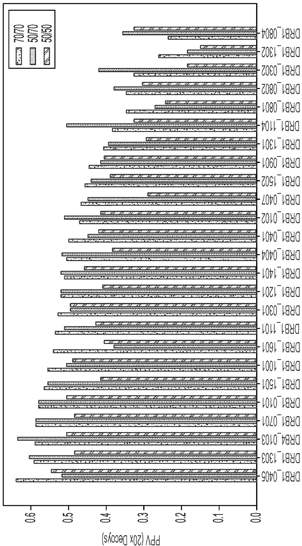
Allele FIG. 5
