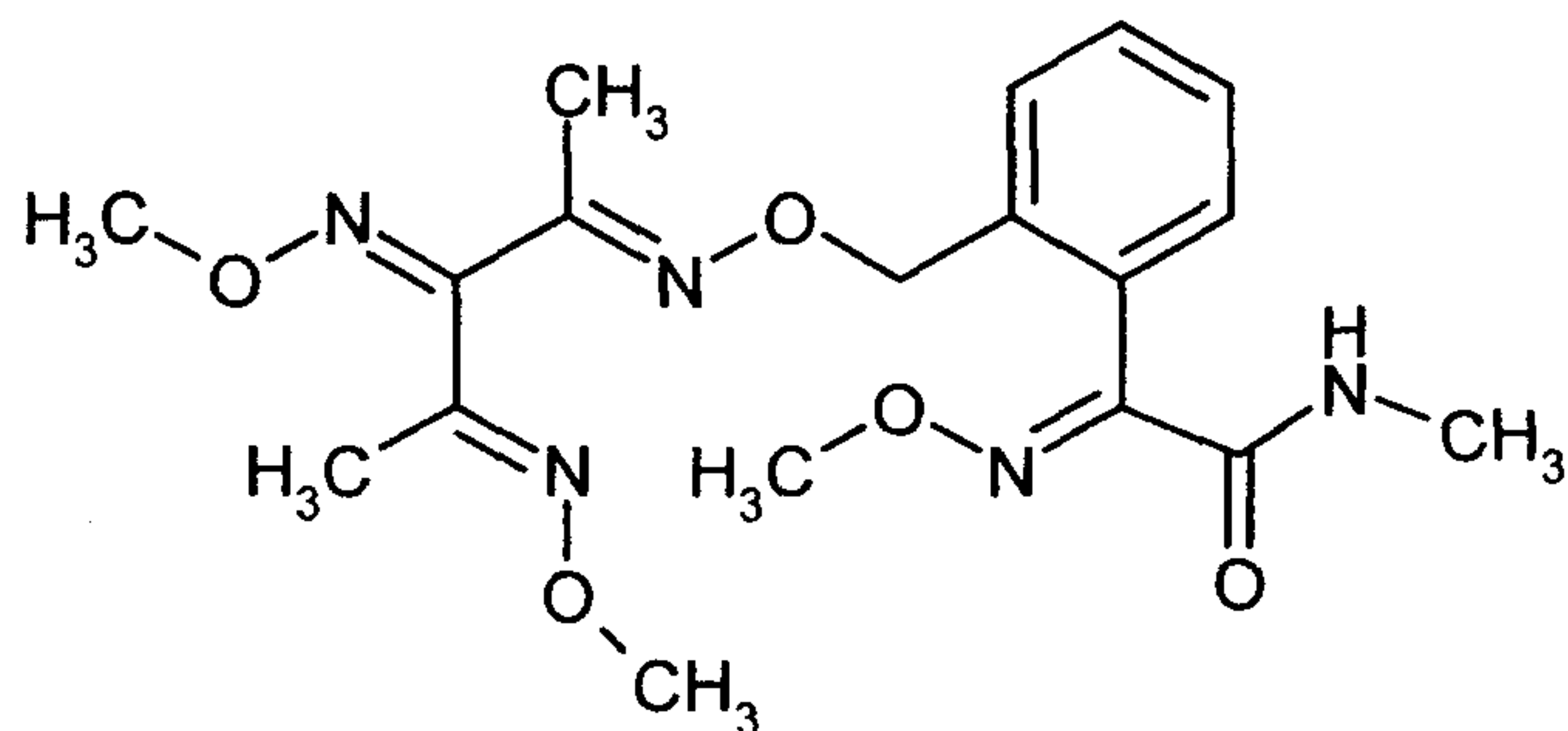
(Orysastrobin)
