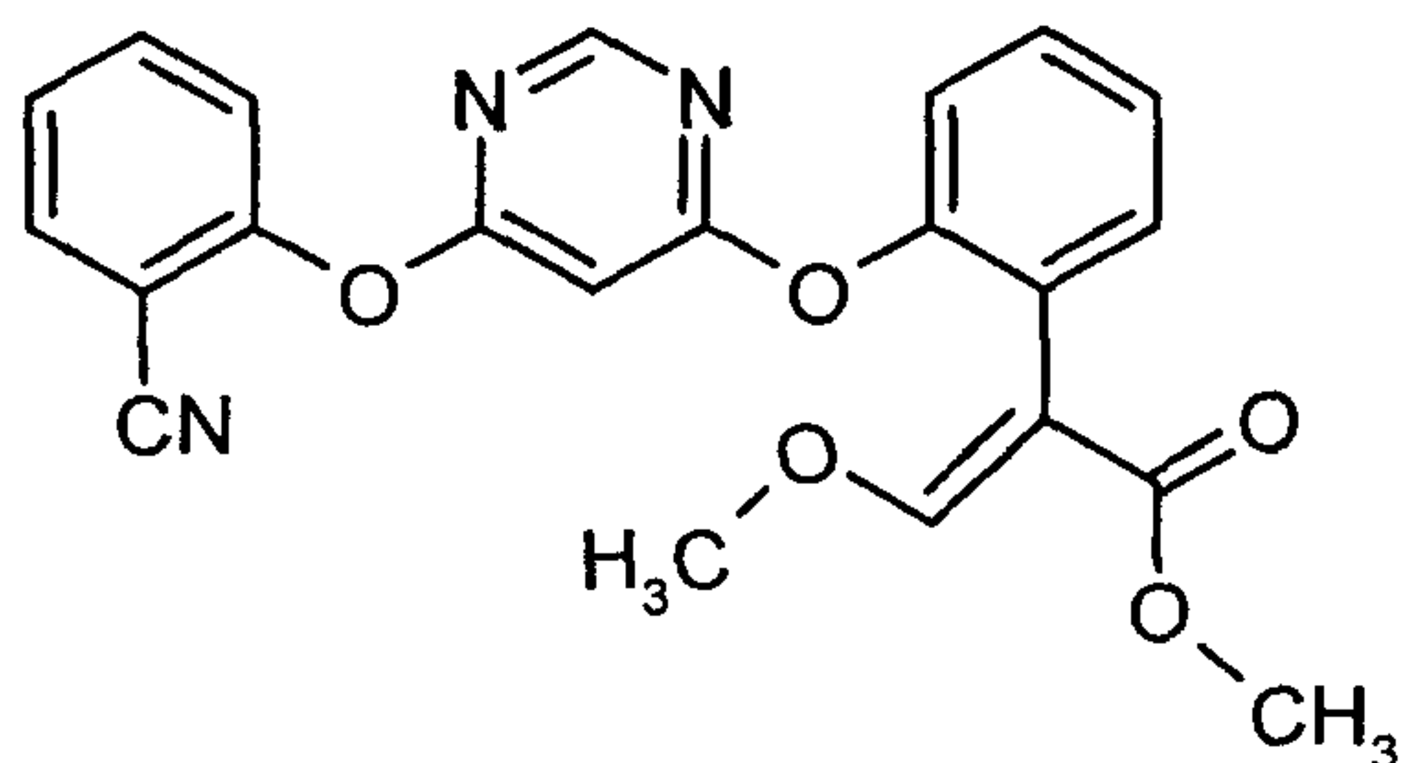
(Azoxystrobin)
