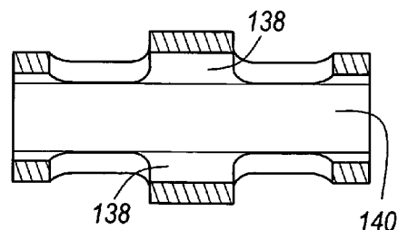
FIG. 14C SECTION B B
