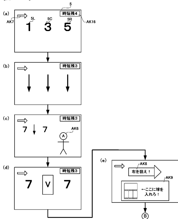
【图12-35】
