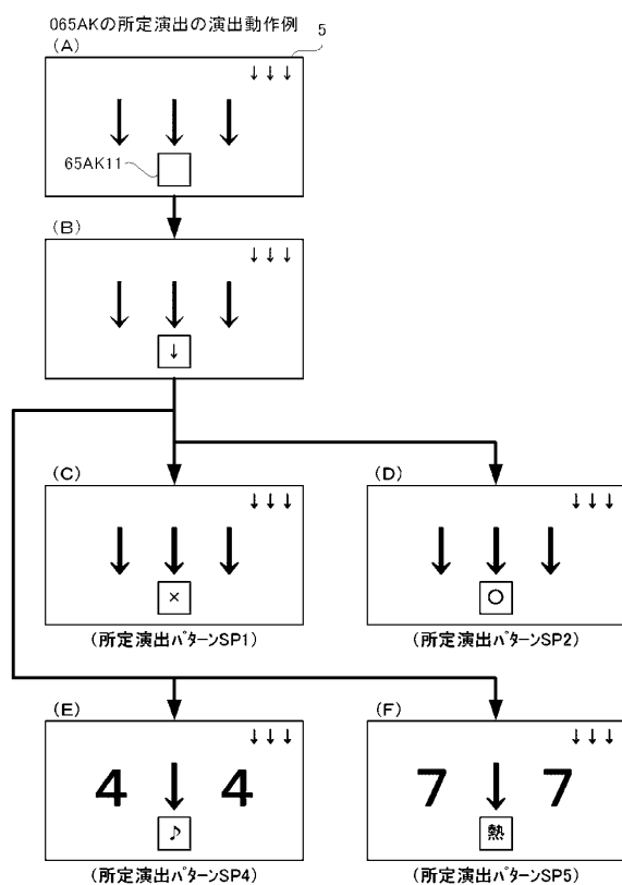
【图13-12】
