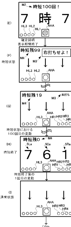
【图 11-33】
