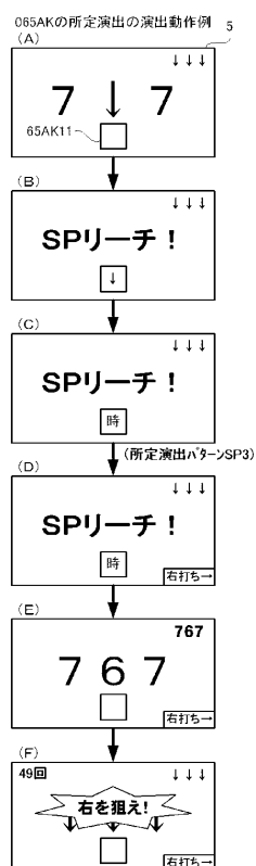
【图13-14】
