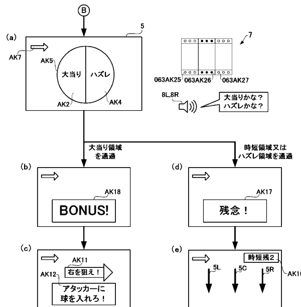
【图12-36】
