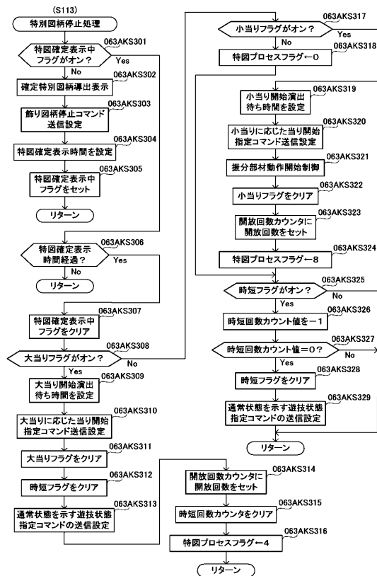
【图12-20】
