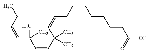
11,11,14,14-Tetramethyl-octadeca-9,12,15-trienoic acid
