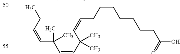
11,11,14,14-Tetramethyl-octadeca-9,12,15-trienoic acid
