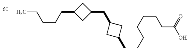
8-[3-(Pentyl-cyclobutylmethyl)-cyclobutyl]-octanoic acid
