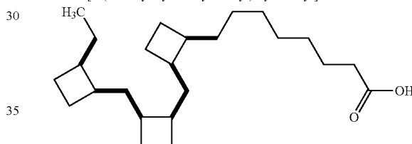
8-[2-[2-(2-Ethyl-cyclobutylmethyl)-cyclobutylmethyl]-cyclobutyl]-octanoic acid
