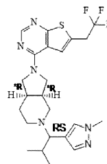
Соединение 78
