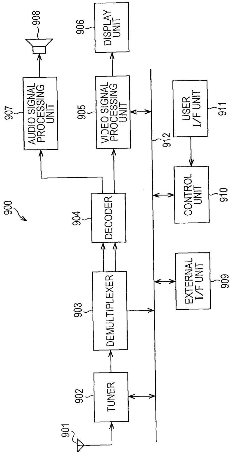
FIG. 28
