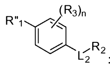
Formula (IVA).
