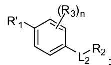
Formula (VIIA).
