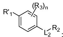
Formula (VIIA).
