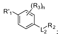
Formula (VA).
