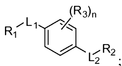
Formula (IA).
