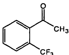
[Chem. 6]
