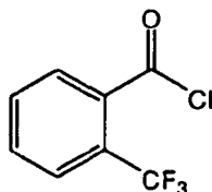
[Chem. 3]
