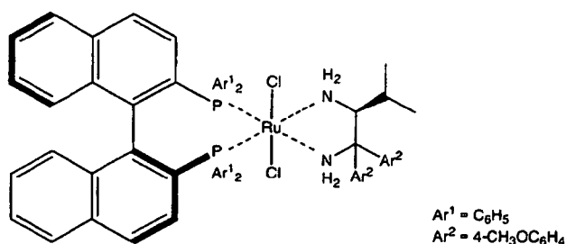
[Chem. 5]
