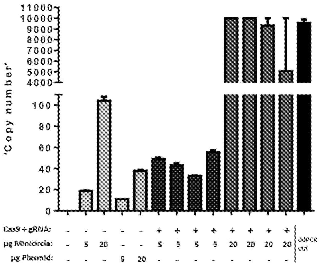
FIG. 80 mTCRb ddPCR - Day 4
