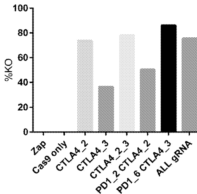
FIG. 26 A CTLA4 KO
