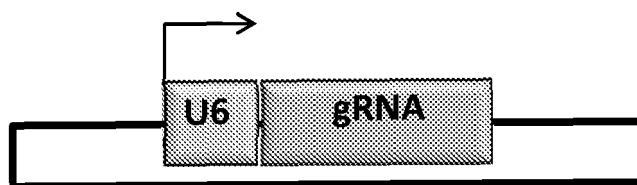
HPRT Guide RNA (4.4 kb)
