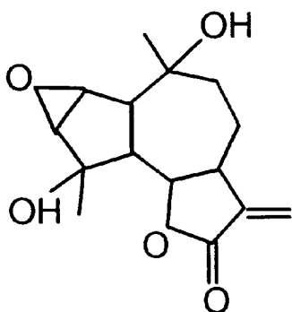
ANOBIN 19
