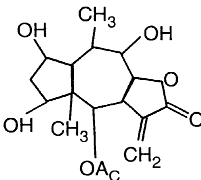
GAIGRANIN 21
