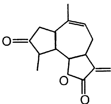
GLABELLIN 17
