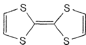
TTF
