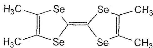
TMTSF
