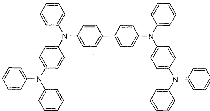
TPD232
