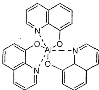
Alq
