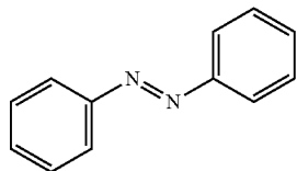
(E)-diphenyldiazene, (E)-Azobenzene
